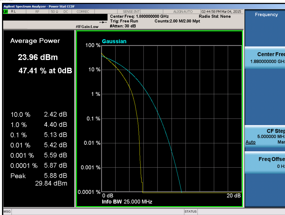
Plot 6-124. PAR Plot (Band 2 – 15.0MHz QPSK – RB Size 75)
