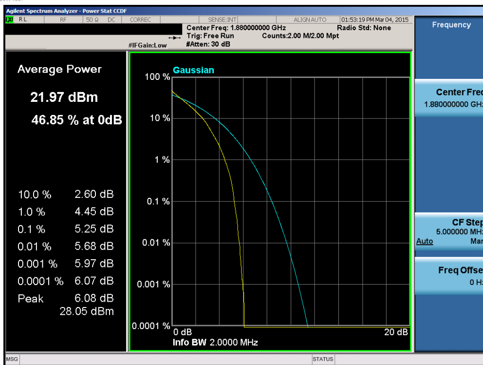
Plot 6-116. PAR Plot (Band 2 – 1.4MHz QPSK – RB Size 6)
