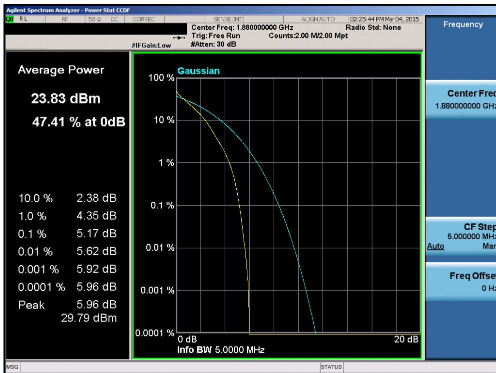
Plot 6-120. PAR Plot (Band 2 – 5.0MHz QPSK – RB Size 25)
