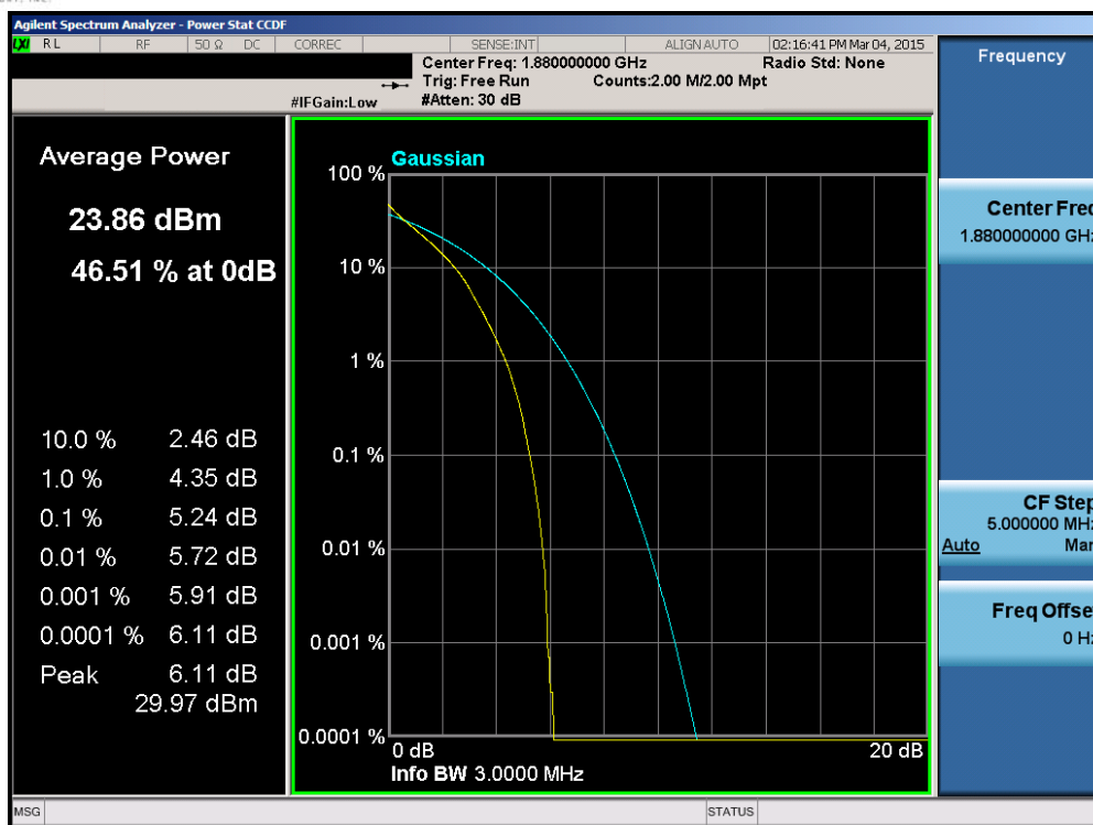
Plot 6-118. PAR Plot (Band 2 – 3.0MHz QPSK – RB Size 15)
