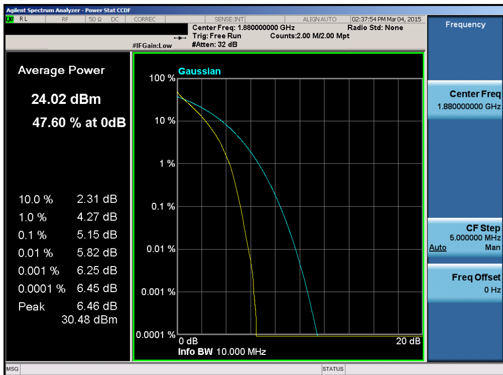
Plot 6-122. PAR Plot (Band 2 – 10.0MHz QPSK – RB Size 50)
