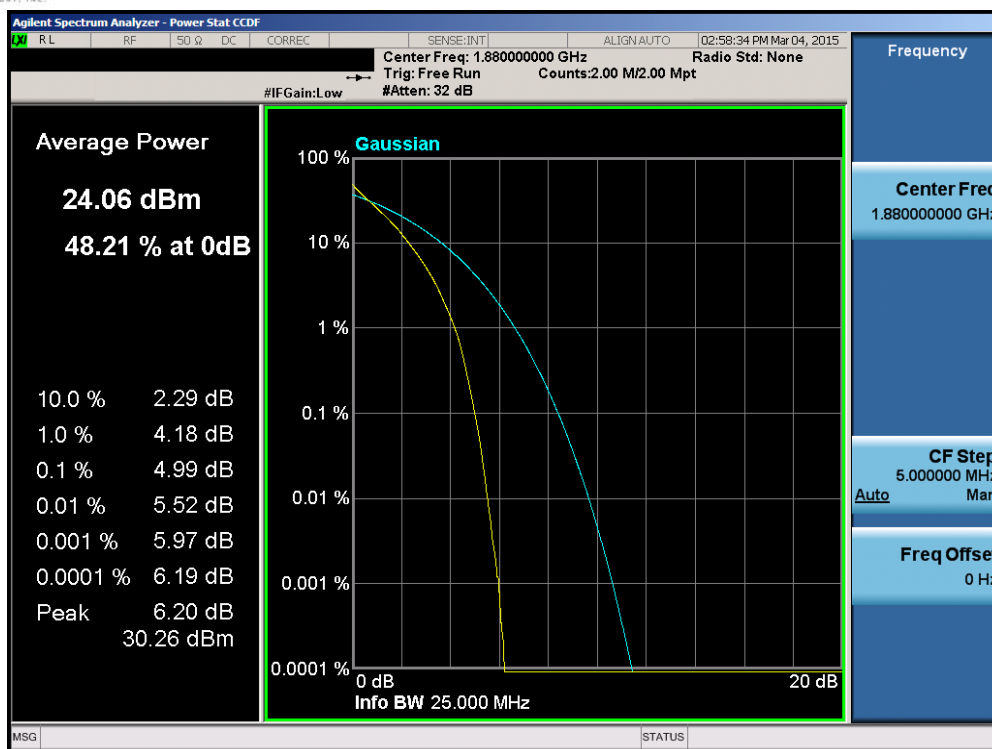
Plot 6-126. PAR Plot (Band 2 – 20.0MHz QPSK – RB Size 100)
