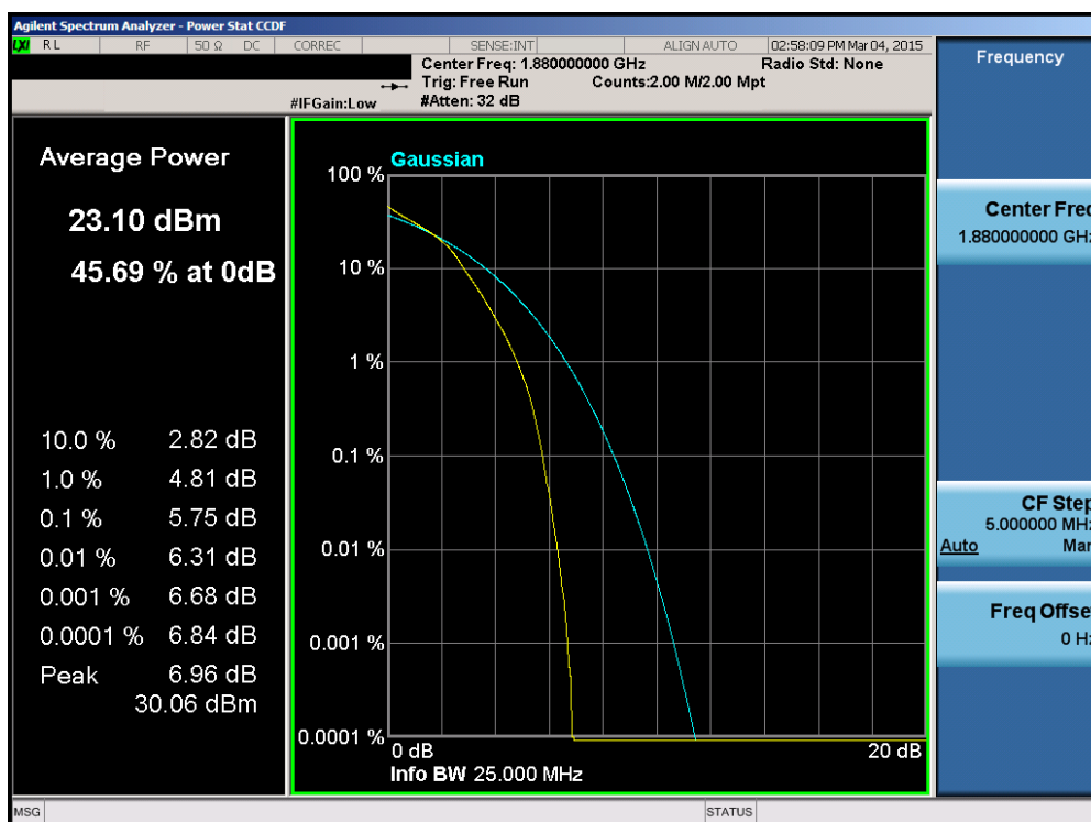
Plot 6-127. PAR Plot (Band 2 – 20.0MHz 16-QAM – RB Size 100)
