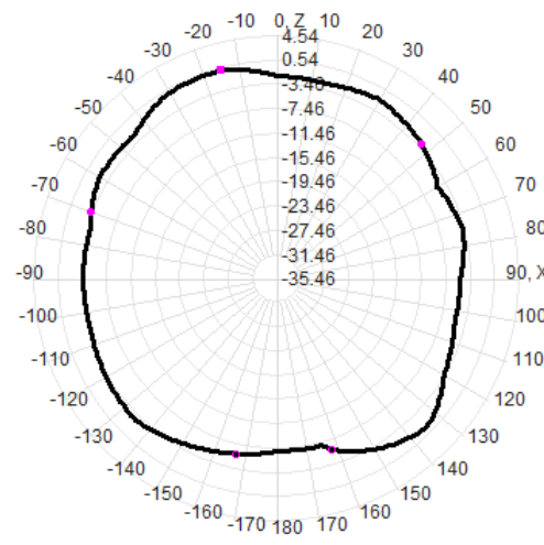
5G phi=0deg
