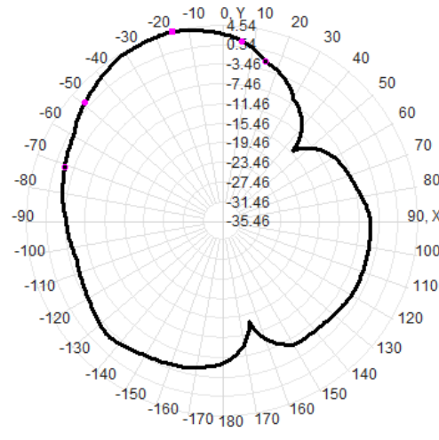
5G theta=90deg
