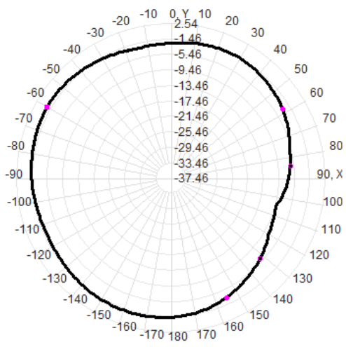
2.4G theta=90deg
