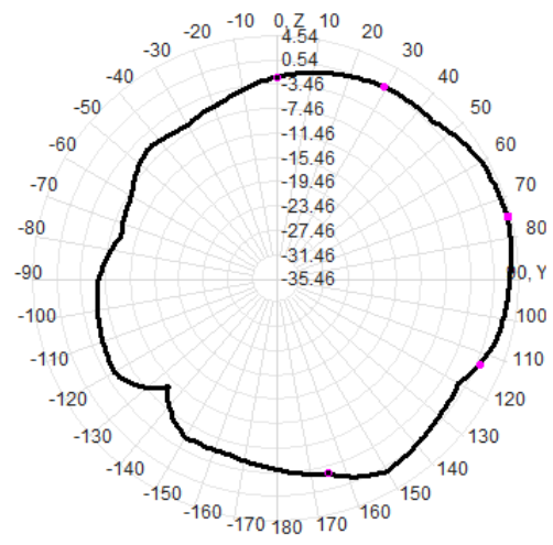
5G phi=90deg
