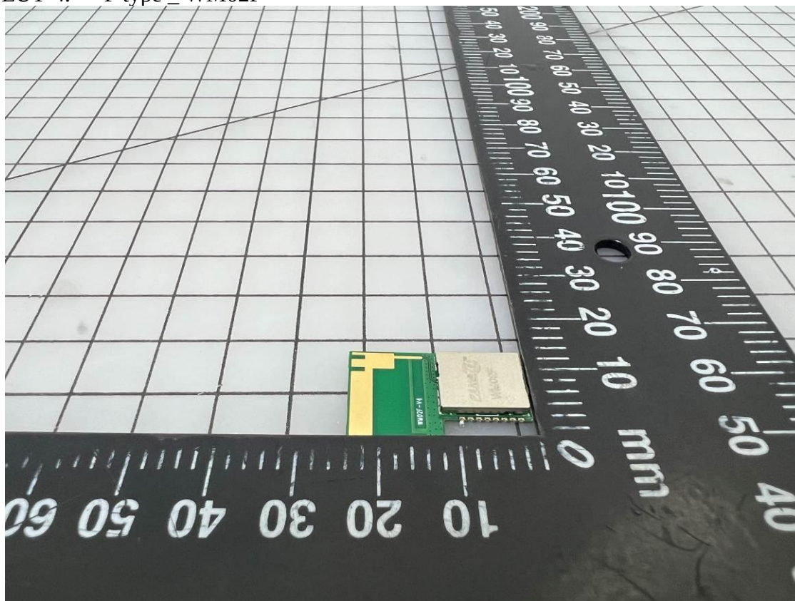
EUT-4. F type _ WM02F
