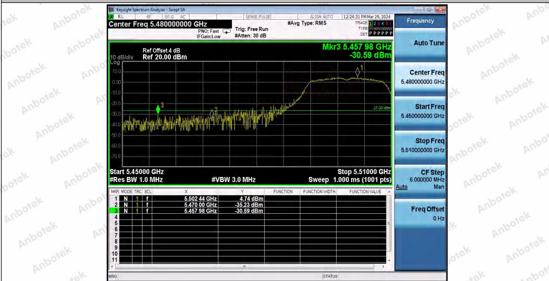
11AC20MIMO_Ant1_Low_5500
