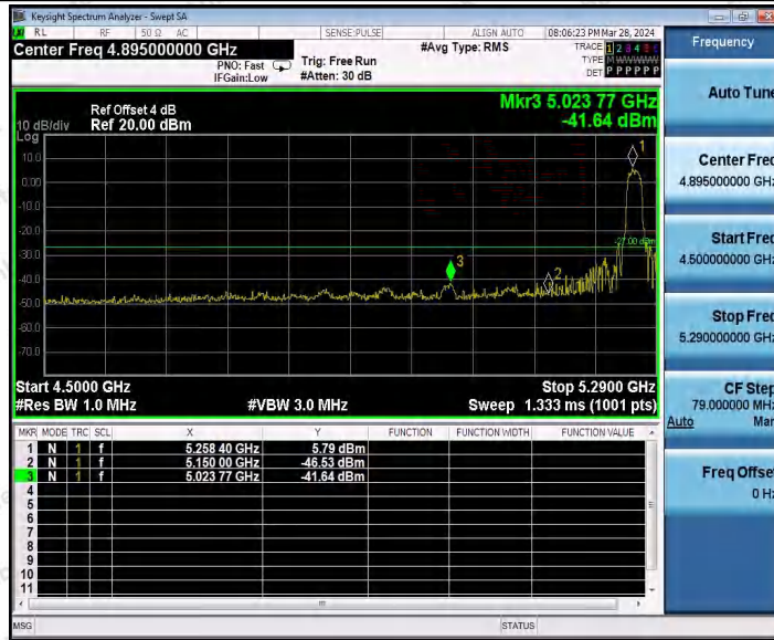
11AC20MIMO_Ant2_Low_5260
