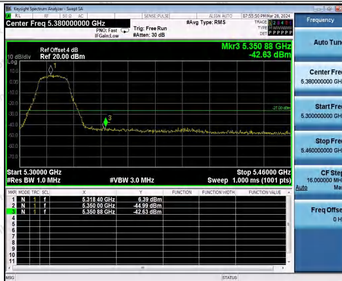
11N20MIMO_Ant2_High_5320
