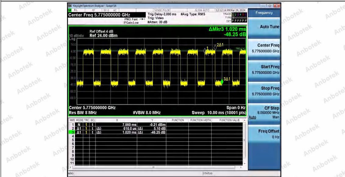
11AX80MIMO_Ant2_5775
