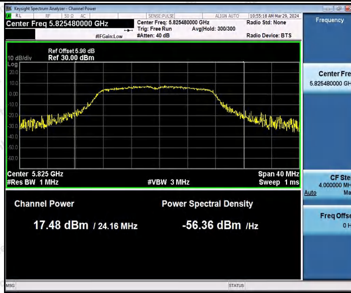
11A_Ant2_5825
