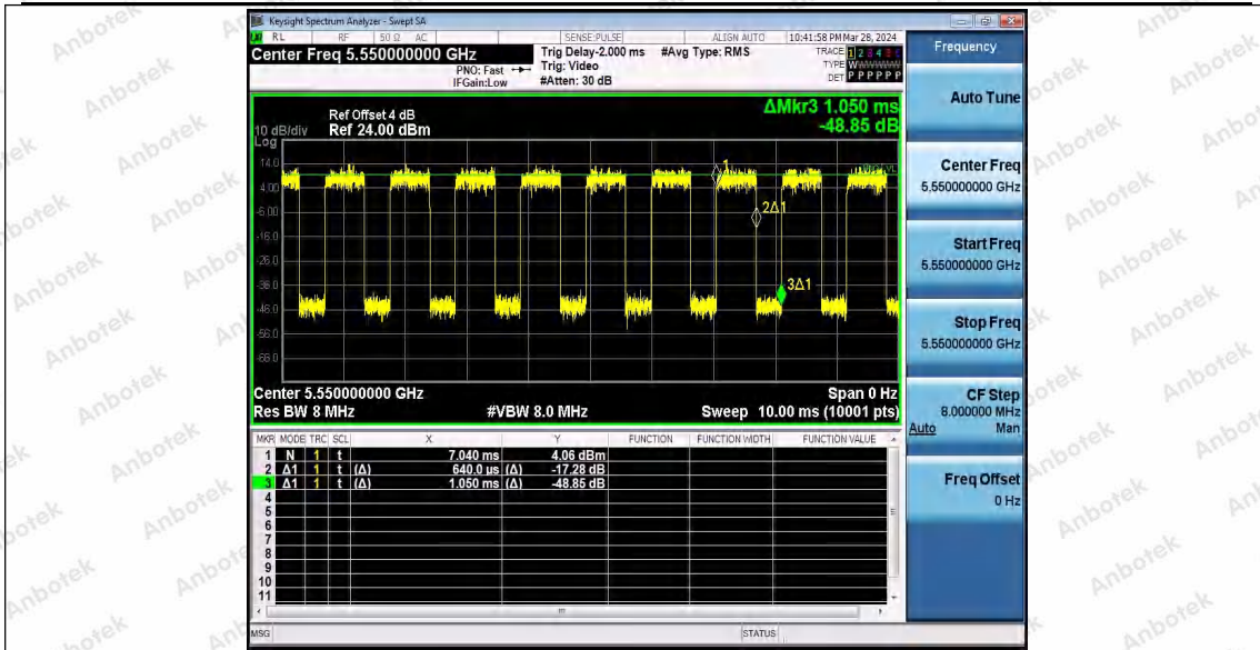
11AX40MIMO_Ant2_5550
