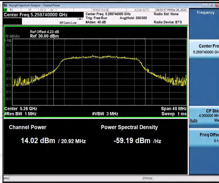
11AC20MIMO_Ant2_5260
