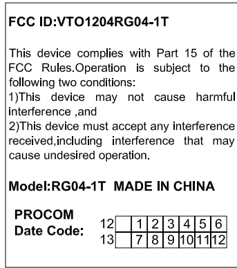
1: 2放大图样
