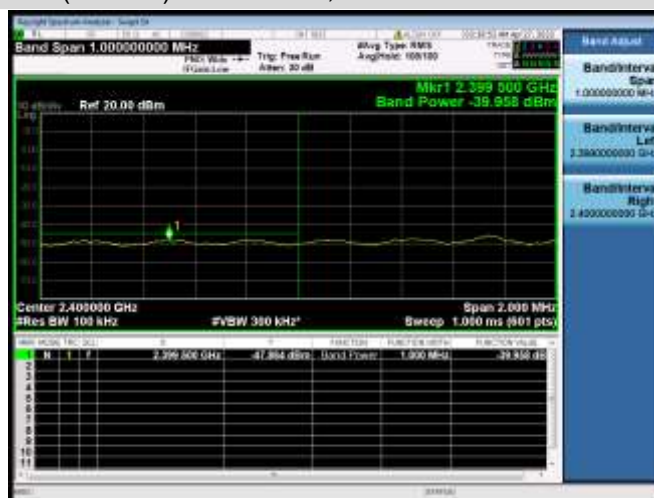
VHT(40 MHz) CHANNEL 4, BAND EDGE
