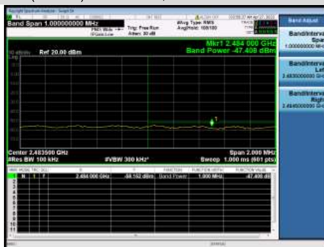
VHT(40 MHz) CHANNEL 8, BAND EDGE
