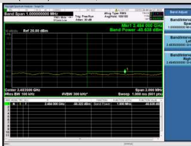
VHT(40 MHz) CHANNEL 7, BAND EDGE
