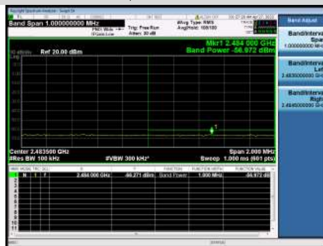
802.11b CHANNEL 9, BAND EDGE
