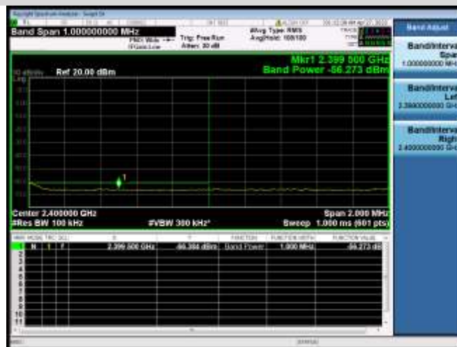
802.11b CHANNEL 5, BAND EDGE
