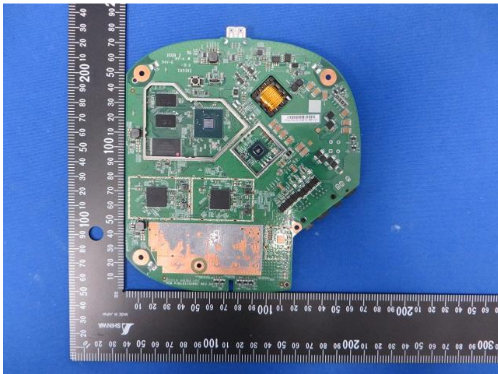
(6) EUT Photo (APIN0514)
