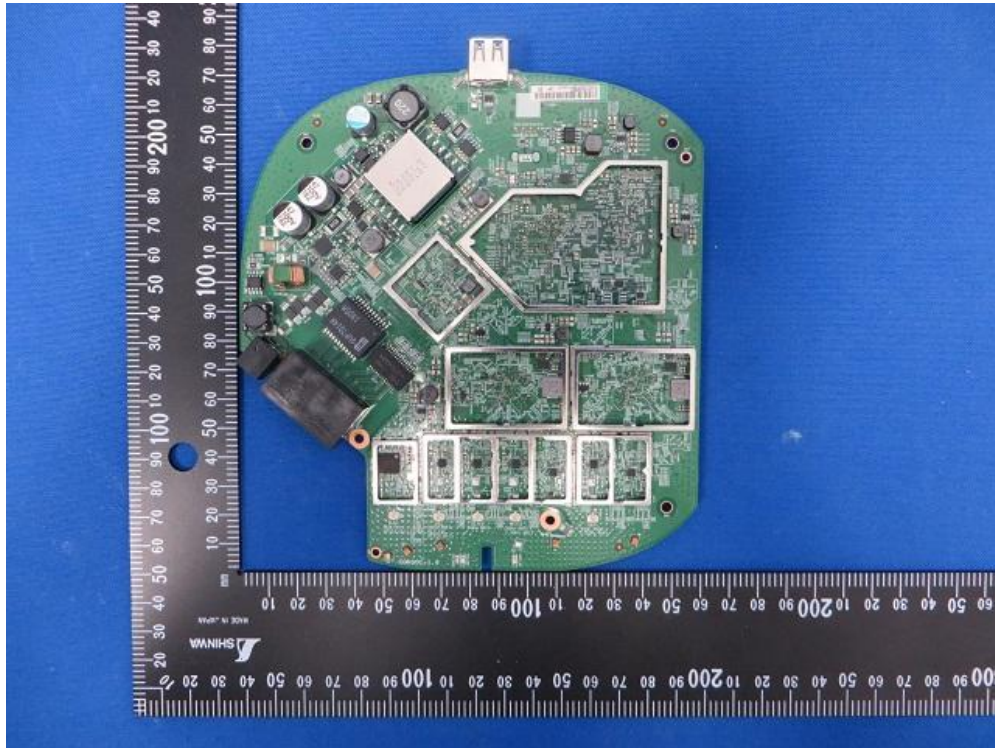
(12) EUT Photo (APIN0514)
