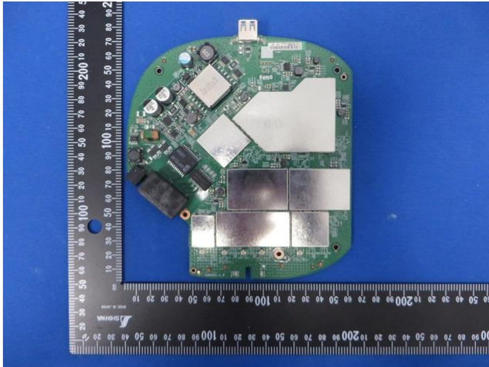
(5) EUT Photo (APIN0514)
