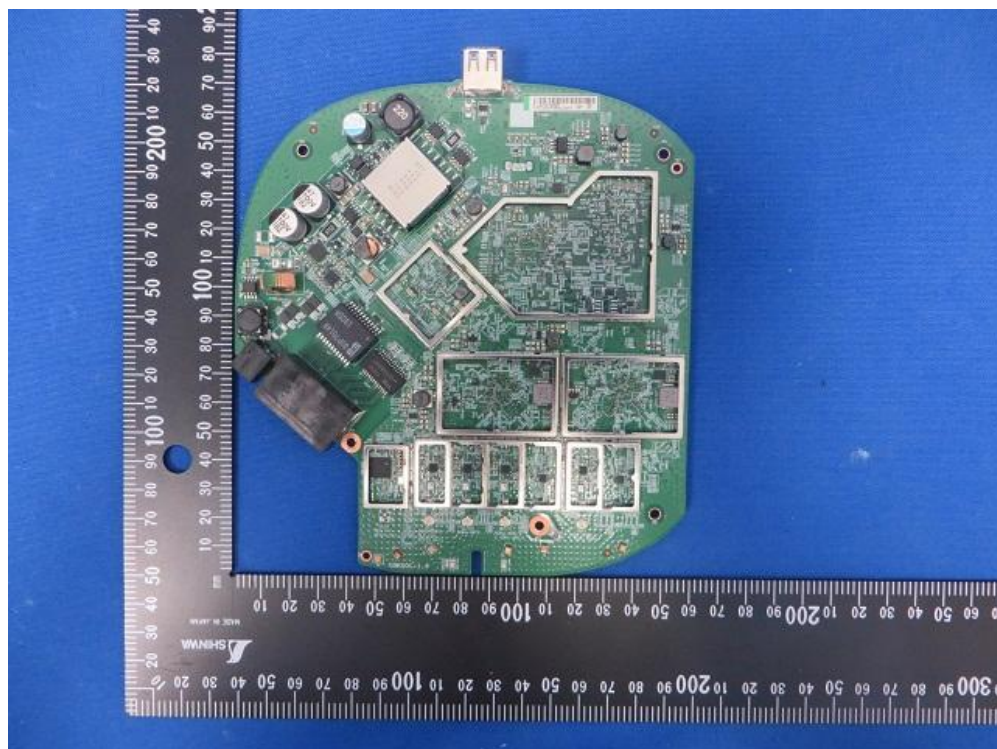
(20) EUT Photo (APIN0515)
