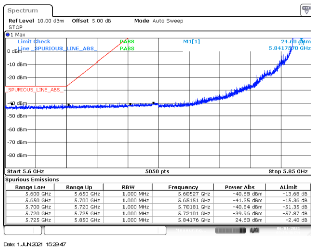
BE-NR-LOW, SISO-A, 802.11ax20-HE0, Ch169
