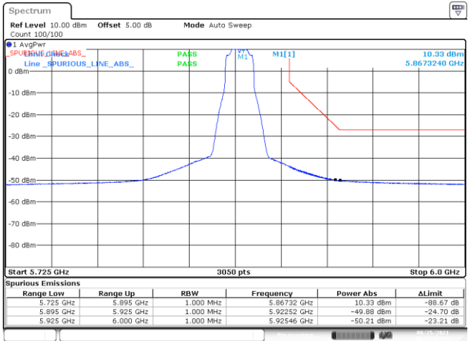
BE-NR-HIGH, SISO-B, 802.11a20-6Mbps, Ch173
