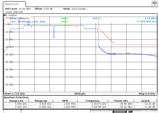
BE-NR-HIGH, MIMO-A, 802.11ax160-HE0, Ch163
