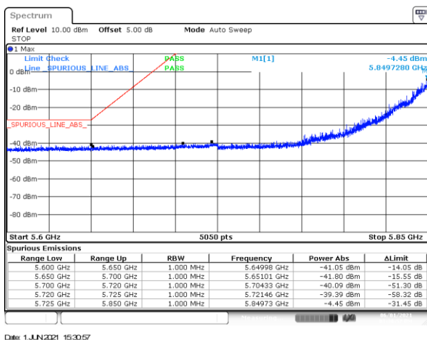
BE-NR-LOW, SISO-A, 802.11ax20-HE0, Ch173
