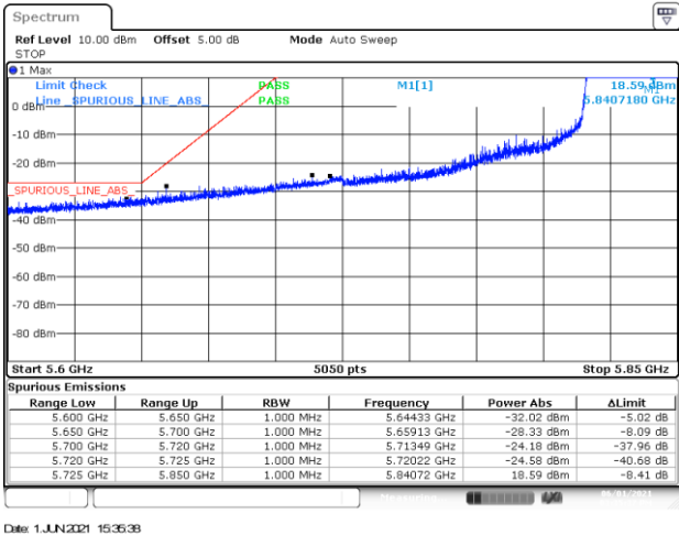
BE-NR-LOW, SISO-A, 802.11ax80-HE0, Ch171
