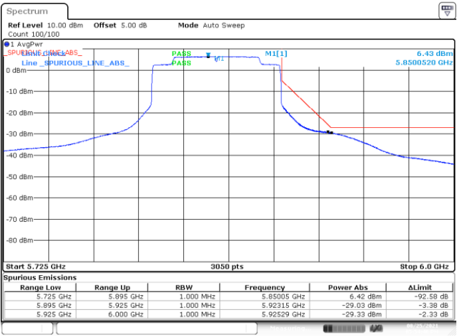
BE-NR-HIGH, SISO-A, 802.11ax160-HE0, Ch163
