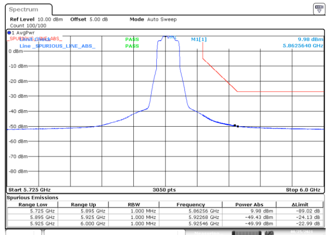
BE-NR-HIGH, SISO-B, 802.11ax20-HE0, Ch173
