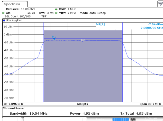
SISO A-802.11ax-20MHz-Ch229-7095MHz-HE0
