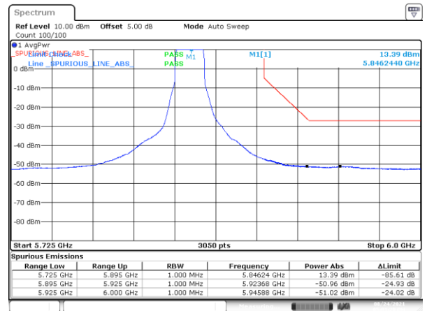
BE-NR-HIGH, MIMO-B, 802.11ax20-HE0, Ch169
