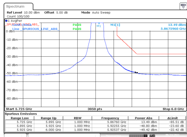
BE-NR-HIGH, MIMO-B, 802.11ax20-HE0, Ch173
