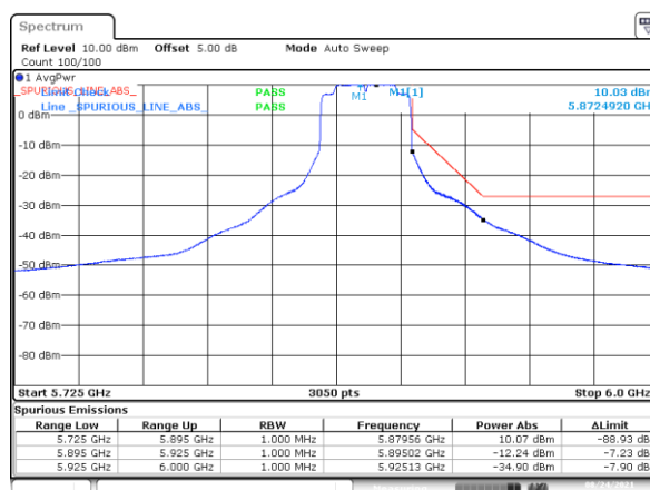
BE-NR-HIGH, SISO-B, 802.11ax40-HE0, Ch175
