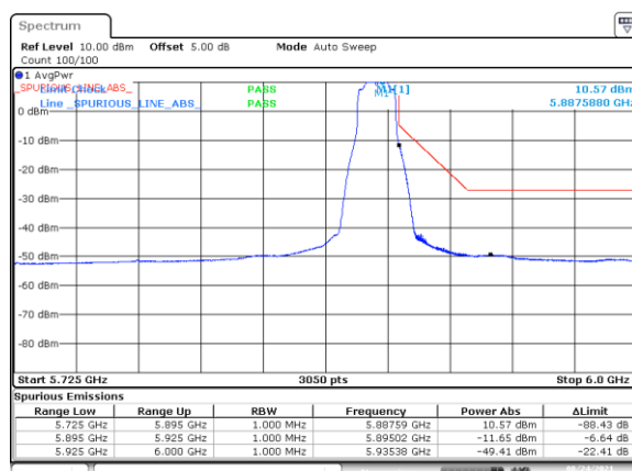
BE-NR-HIGH, SISO-B, 802.11a20-6Mbps, Ch177
