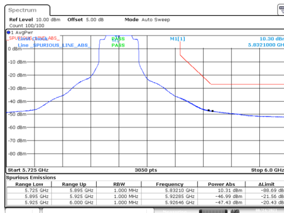
BE-NR-HIGH, SISO-B, 802.11ax40-HE0, Ch167
