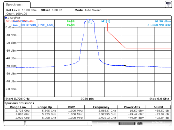
BE-NR-HIGH, SISO-A, 802.11a20-6Mbps, Ch173
