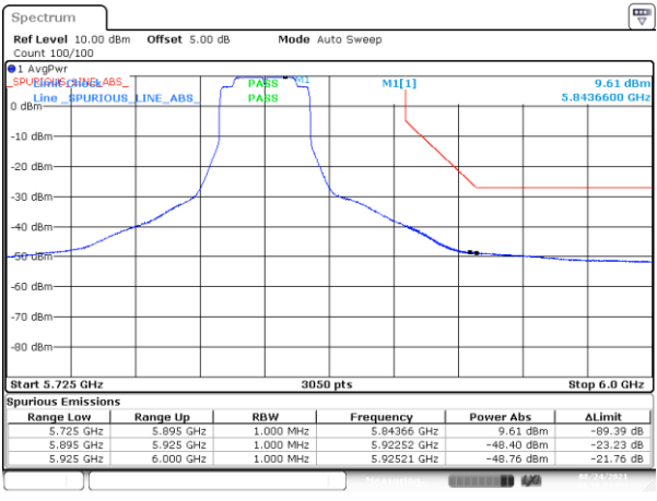
BE-NR-HIGH, SISO-A, 802.11ax40-HE0, Ch167
