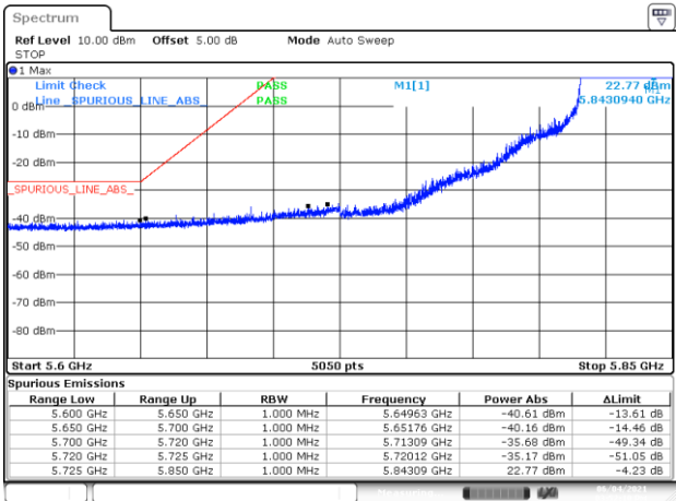
BE-NR-LOW, SISO-A, 802.11ax40-HE0, Ch167
