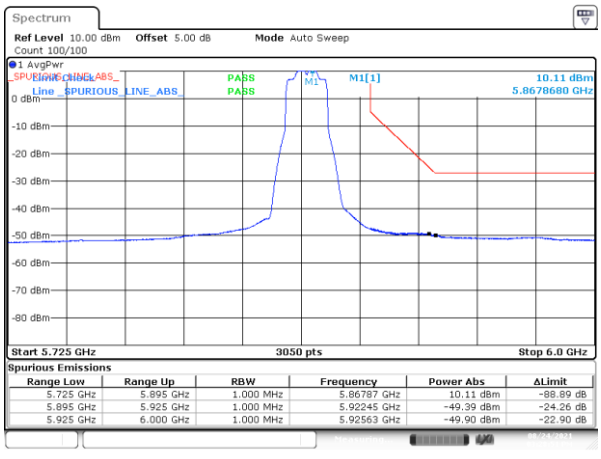
BE-NR-HIGH, SISO-A, 802.11ax20-HE0, Ch173
