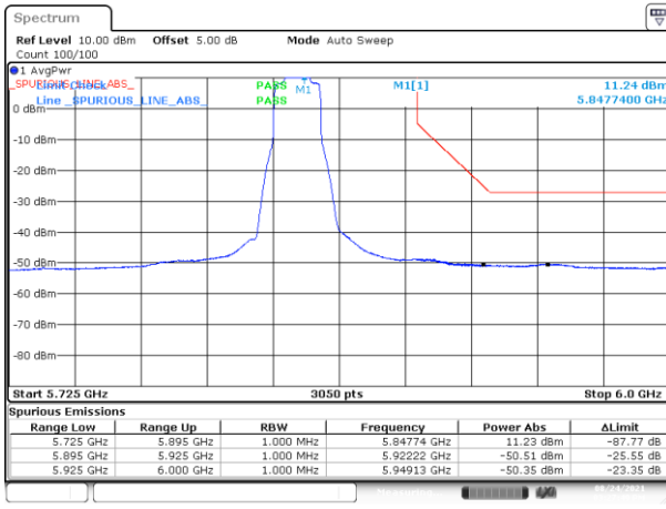
BE-NR-HIGH, SISO-A, 802.11ax20-HE0, Ch169
