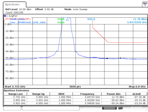
BE-NR-HIGH, SISO-A, 802.11a20-6Mbps, Ch169
