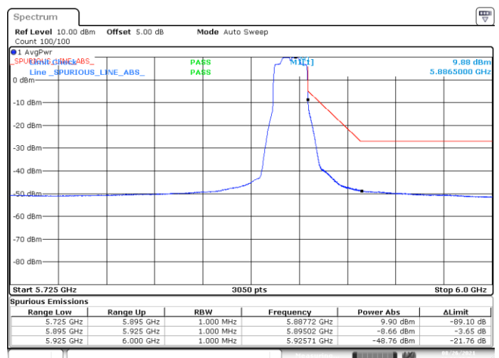
BE-NR-HIGH, SISO-B, 802.11ax20-HE0, Ch177
