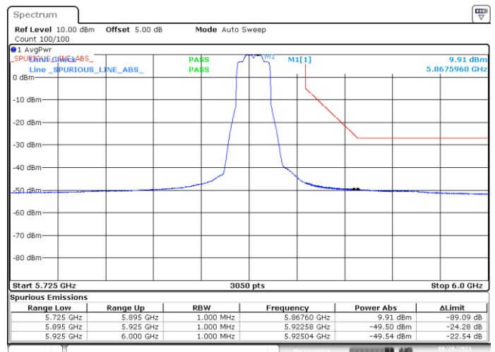
BE-NR-HIGH, SISO-B, 802.11ax20-HE0, Ch173
