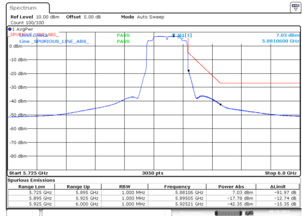
BE-NR-HIGH, MIMO-A, 802.11ax40-HE0, Ch175
