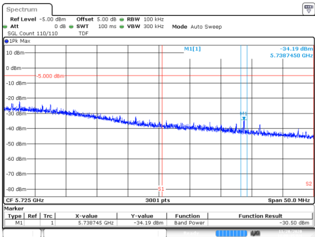
BE-NR-HIGH, DIV 2, 802.11ax40-HE0, Ch134
