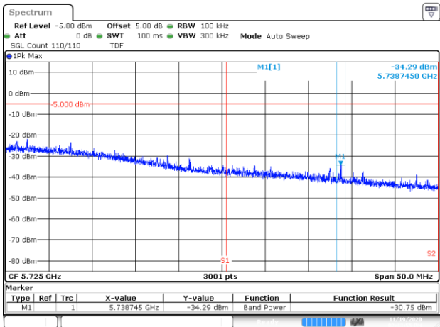
BE-NR-HIGH, DIV 1, 802.11ax40-HE0, Ch134
