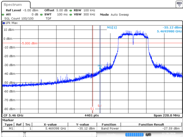
BE-NR-LOW, DIV 2, 802.11n40-HT0, Ch102
