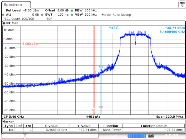
BE-NR-LOW, DIV 1, 802.11n40-HT0, Ch102
