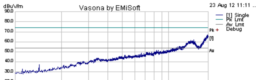
5180 OFDM AVE
