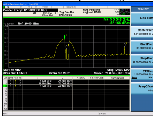
Antenna A
