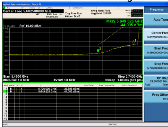
Antenna A
