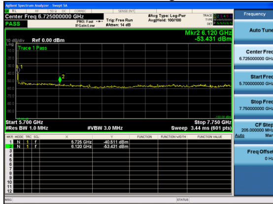
Antenna A
