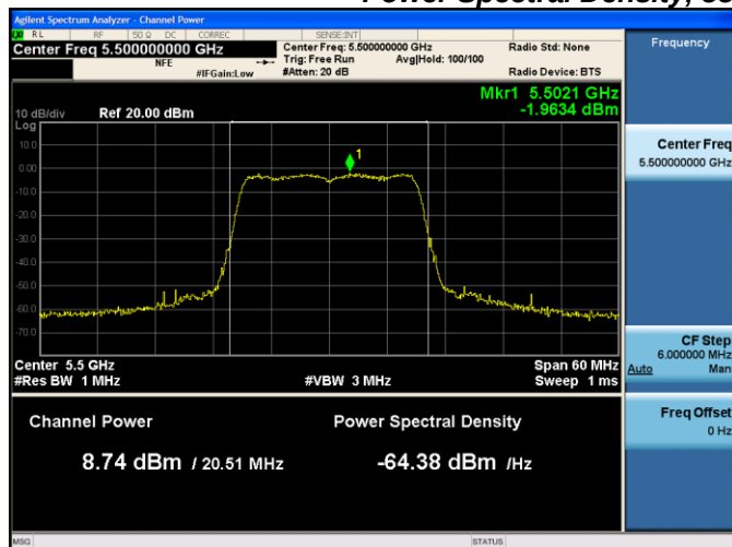
Antenna A
