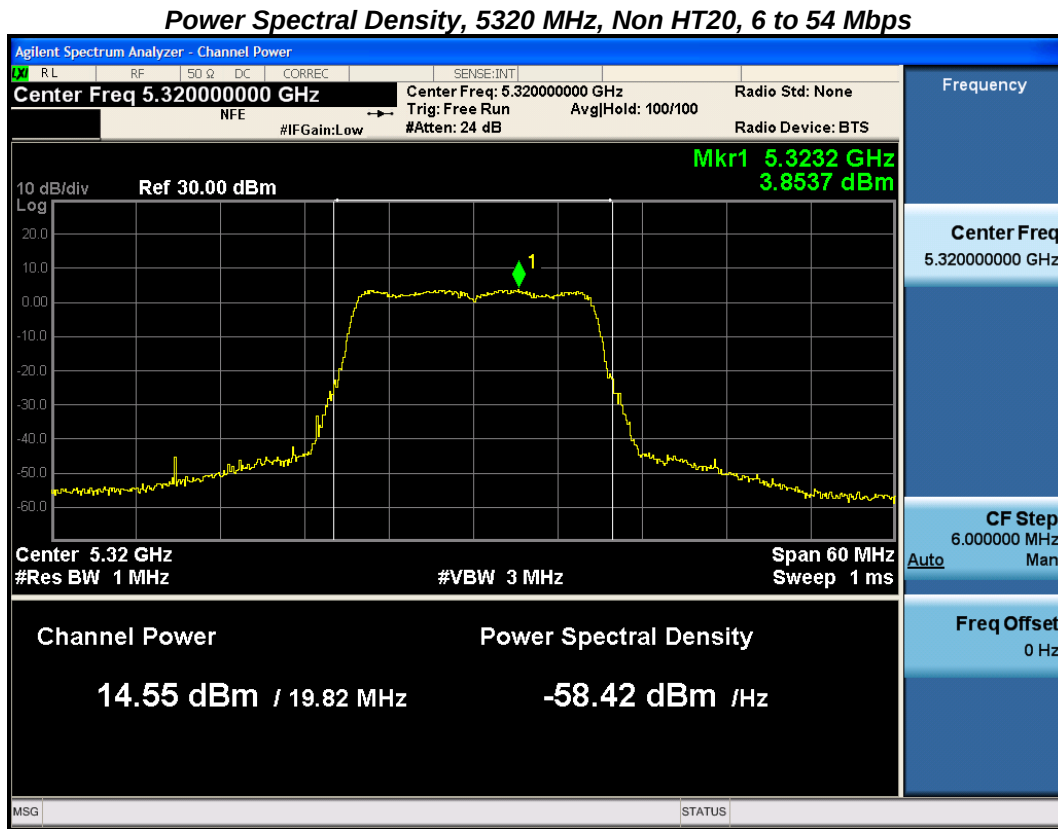
Antenna A
