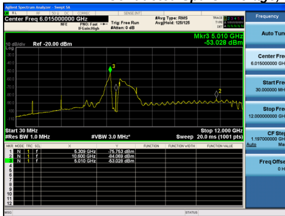
Antenna A
