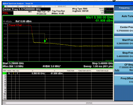
Antenna A
