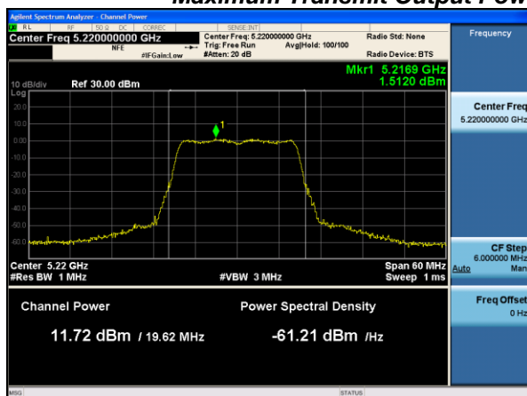
Antenna A
