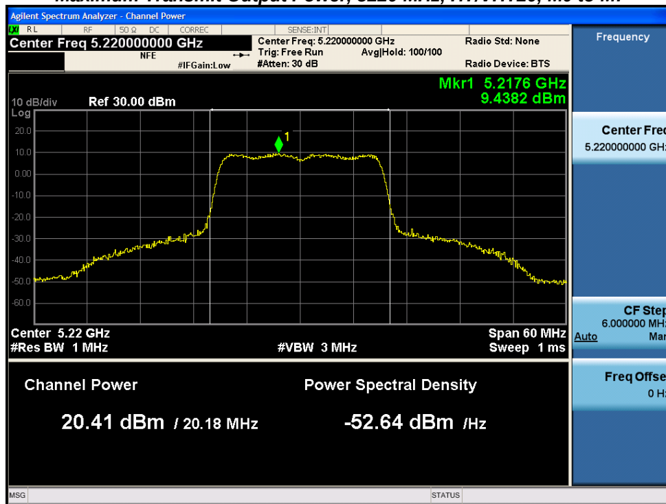
Antenna A
