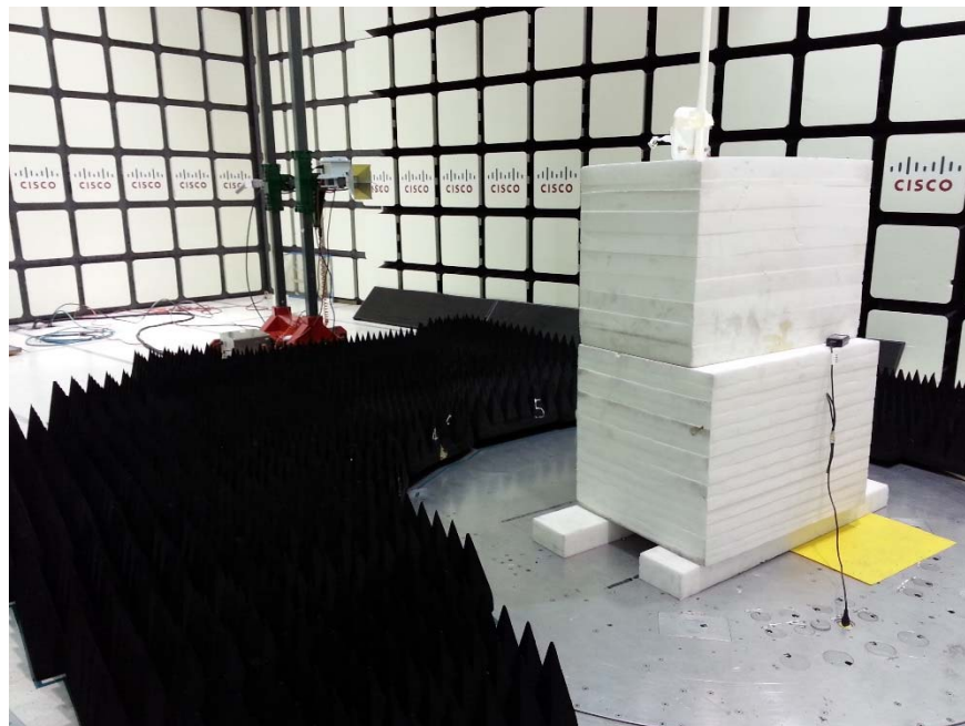
1 – 18GHz Setup
