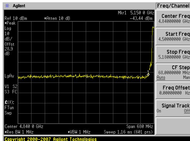
Antenna A
