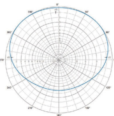
H-Plane | 445 MHz
