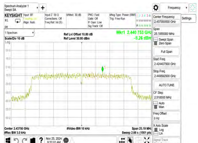
802.11n_20MHz_Chain0_2437MHz
