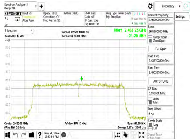
802.11ax_40MHz_Chain0_2462MHz_RU484
