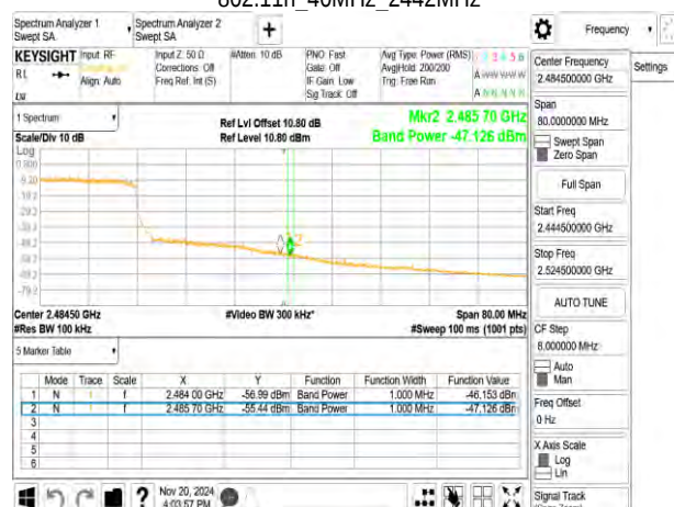
802.11n_40MHz_2442MHz
