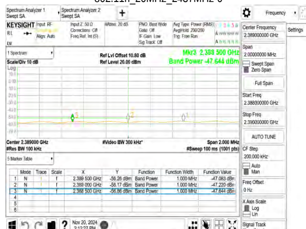
802.11n_20MHz_2437MHz-0
