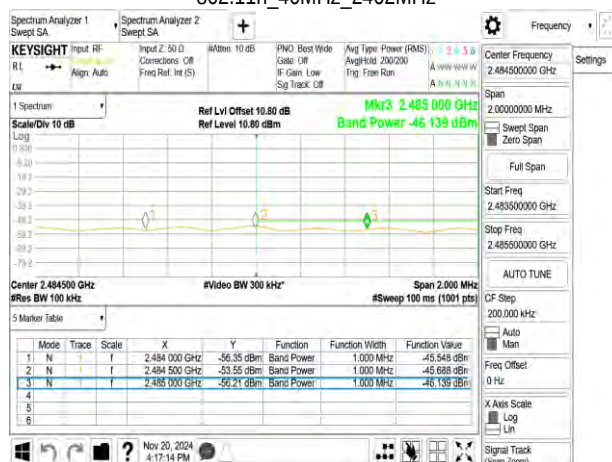
802.11n_40MHz_2462MHz
