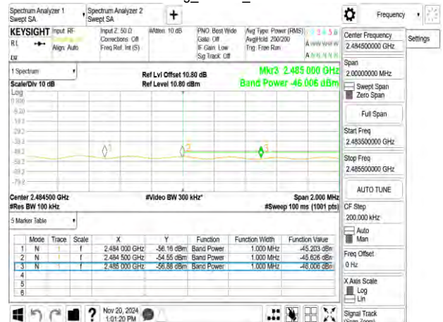
802.11g_20MHz_2472MHz
