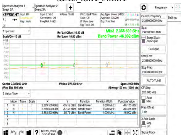
802.11n_20MHz_2422MHz
