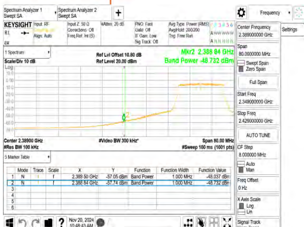
802.11g_20MHz_2422MHz
