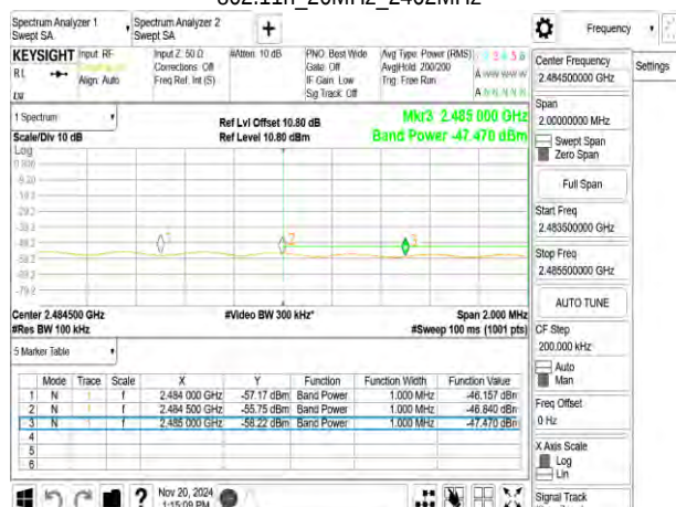
802.11n_20MHz_2462MHz
