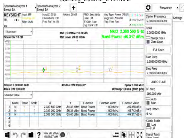
802.11g_20MHz_2417MHz
