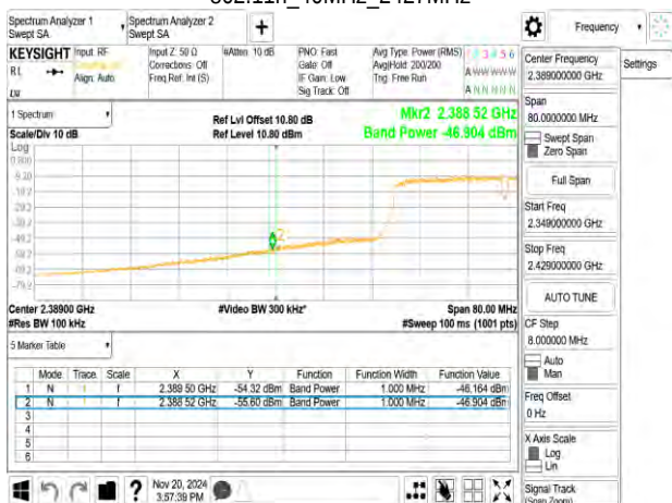
802.11n_40MHz_2427MHz
