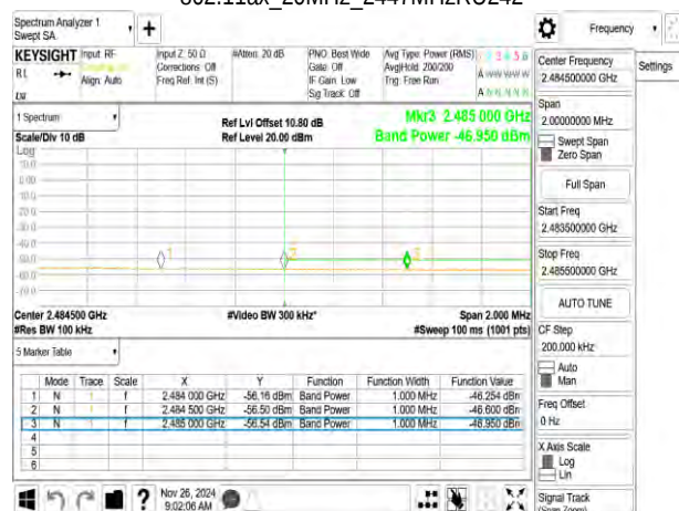
802.11ax_20MHz_2447MHzRU242
