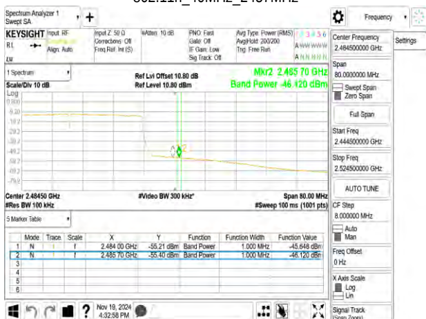
802.11n_40MHz_2457MHz
