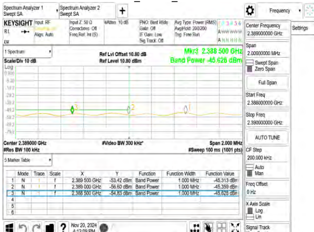
802.11n_40MHz_2422MHz
