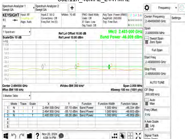
802.11n_40MHz_2447MHz
