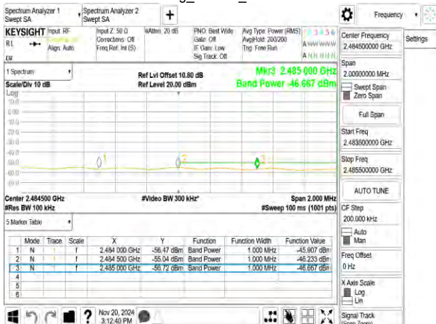
802.11g_20MHz_2457MHz
