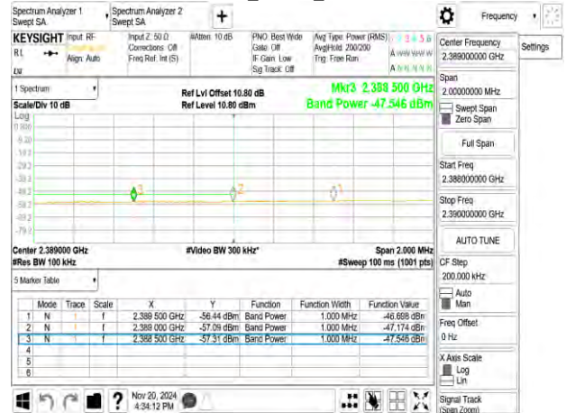
802.11ax_20MHz_2427MHzRU242
