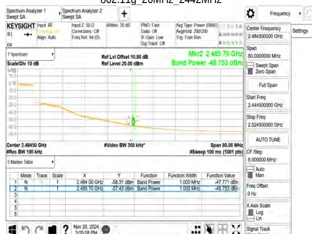
802.11g_20MHz_2442MHz
