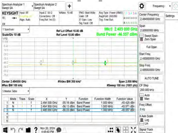
802.11ax_20MHz_2457MHz
