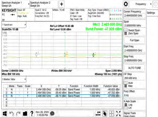
802.11n_20MHz_2472MHz
