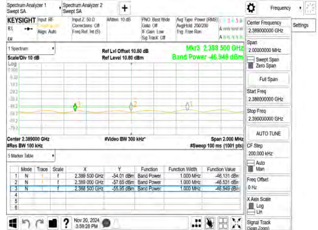
802.11n_40MHz_2432MHz
