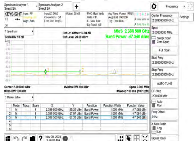
802.11n_40MHz_2437MHz-0
