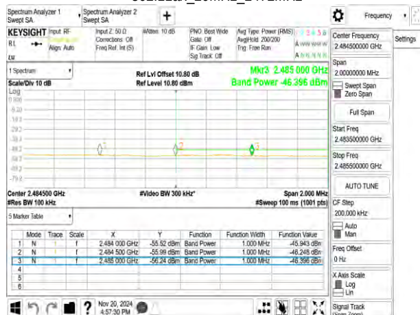
802.11ax_20MHz_2472MHz
