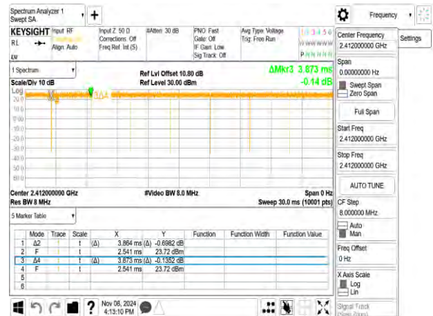
802.11ax_20MHz_Chain0_2412MHz_RU26_0
