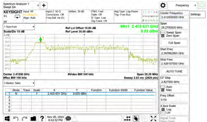
802.11ax_20MHz_Chain0_2412MHz_RU52_37
