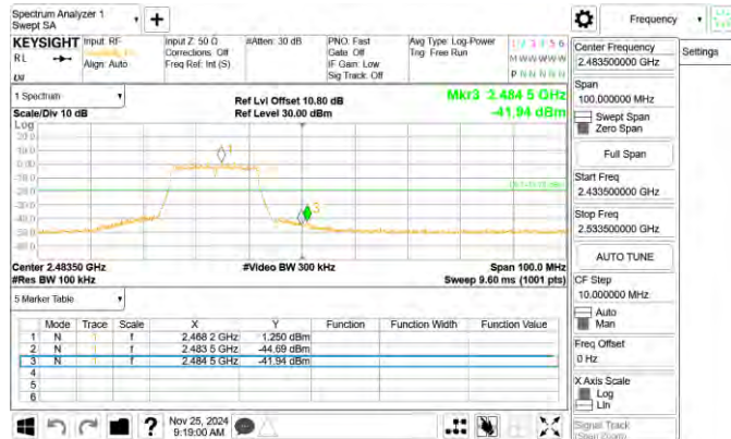
802.11g_20MHz_Chain0_2472MHz
