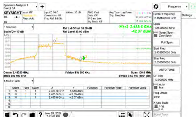
802.11ax_20MHz_Chain0_2462MHz_RU242.
