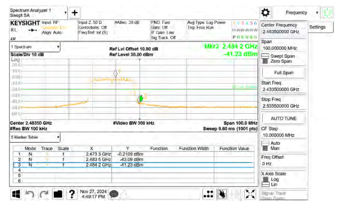
802.11n_20MHz_Chain0_2472MHz
