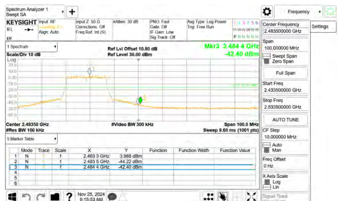
802.11g_20MHz_Chain0_2462MHz
