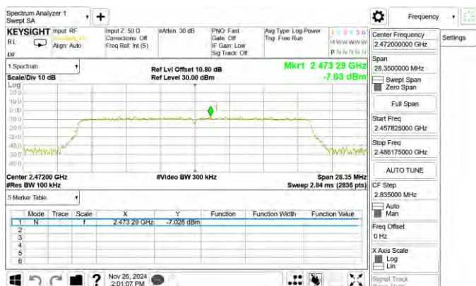
802.11ax_20MHz_Chain0_2472MHz_RU242
