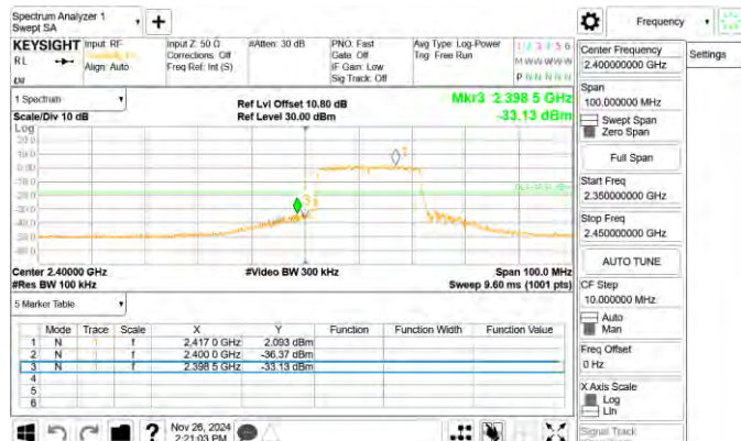
802.11ax_20MHz_Chain0_2412MHz_RU26_0
