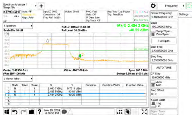
802.11ax_40MHz_Chain0_2457MHz_RU484
