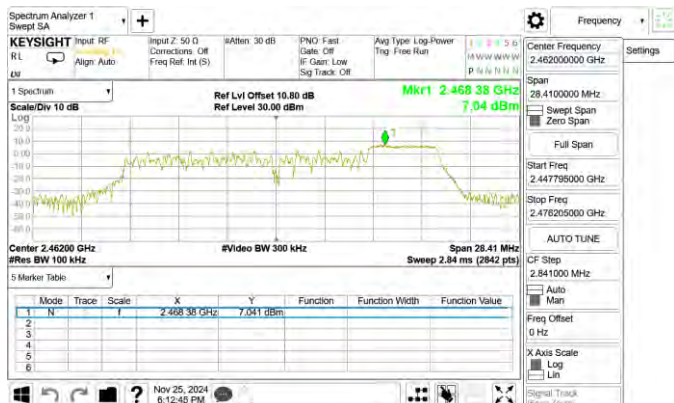
802.11ax_20MHz_Chain0_2462MHz_RU52_40
