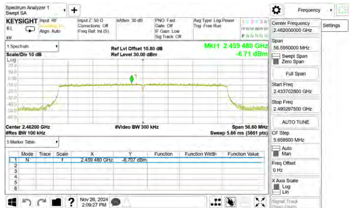
802.11ax_40MHz_Chain0_2462MHz_RU484
