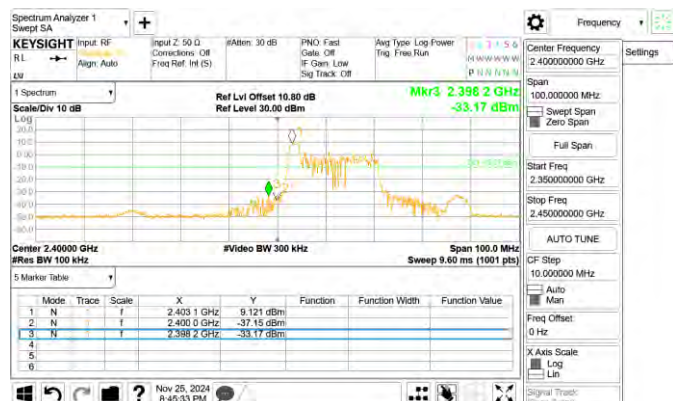
802.11ax_20MHz_Chain0_2412MHz_RU52_37
