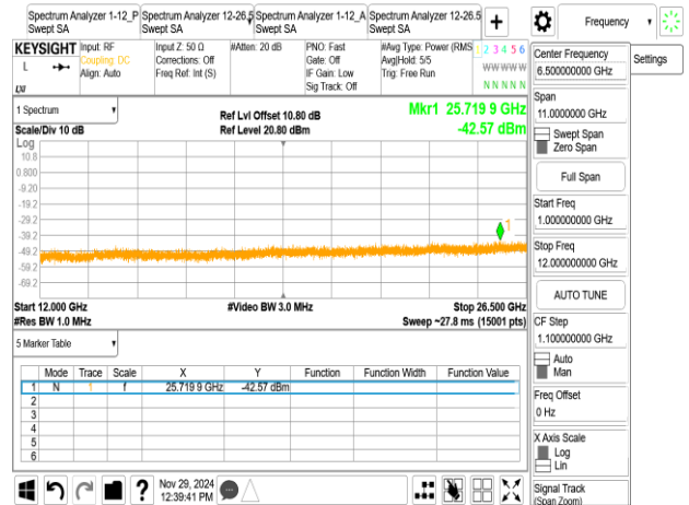
BLE_1M_2440MHz
