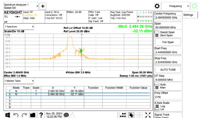
CBE_BLE_500k_2480MHz
