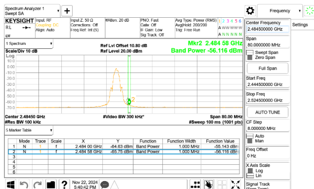
CBE_BLE_2M_2480MHz
