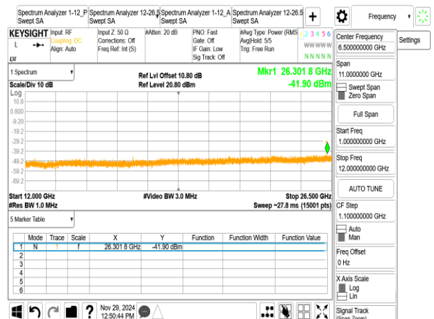
BLE_1M_2480MHz
