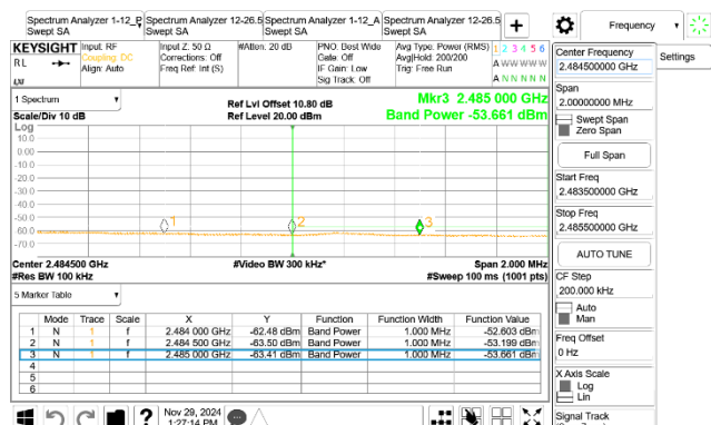
CBE_BLE_1M_2480MHz
