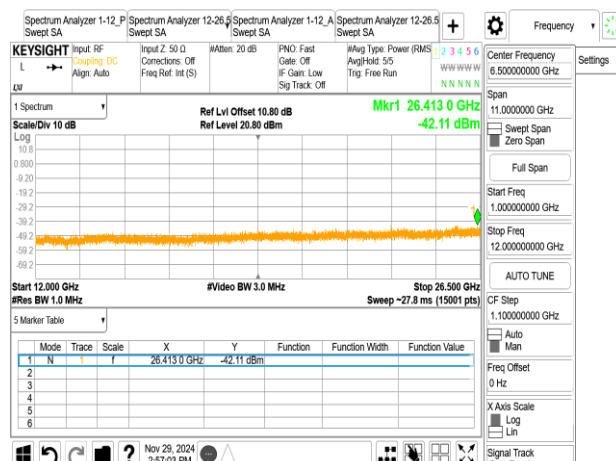
BLE 500k 2480MHz
