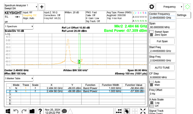
CBE_BLE_500k_2480MHz
