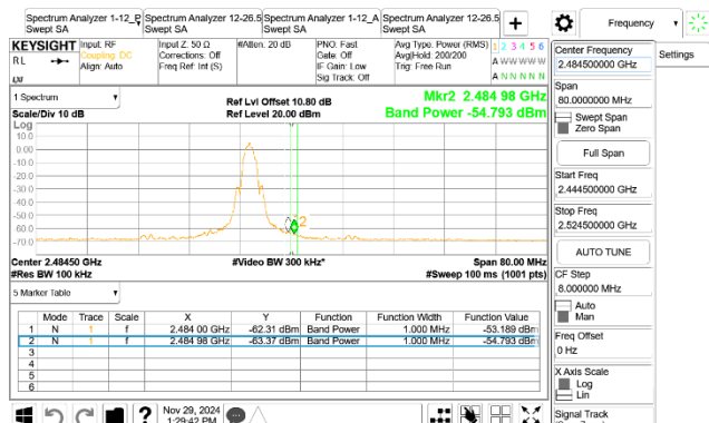
CBE_BLE_2M_2480MHz
