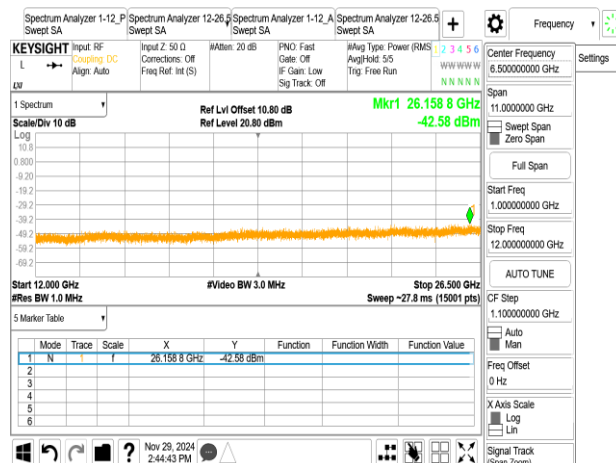
BLE 500k 2442MHz
