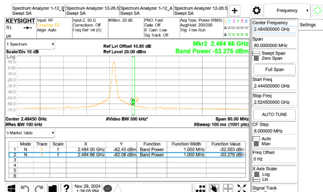
CBE_BLE_1M_2480MHz
