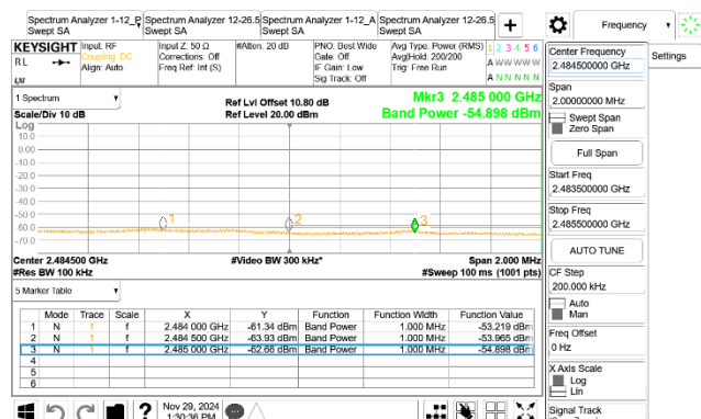
CBE_BLE_2M_2480MHz
