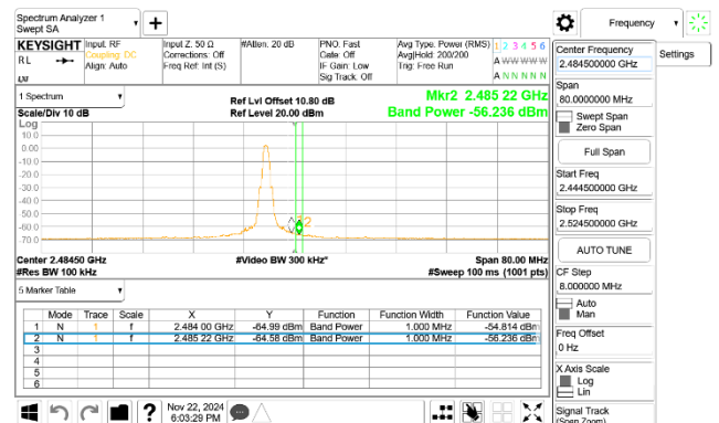
CBE_BLE_500k_2480MHz
