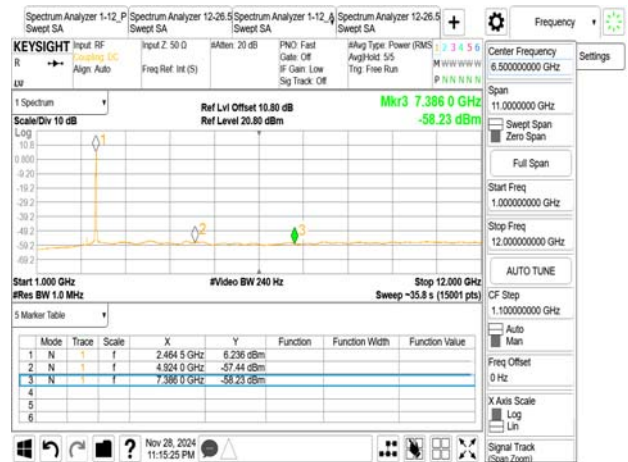
802.11ax_20MHz_2462MHz_RU242
