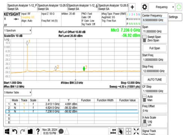
802.11g_20MHz_2412MHz
