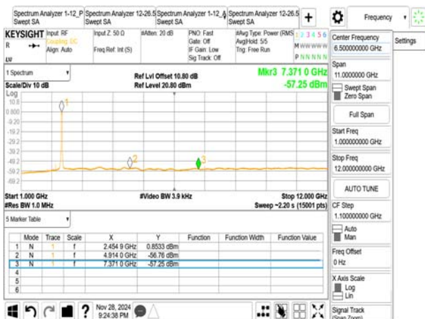
802.11n_40MHz_2462MHz
