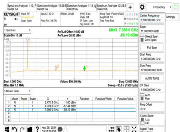
802.11ax_20MHz_2462MHz_RU26_8
