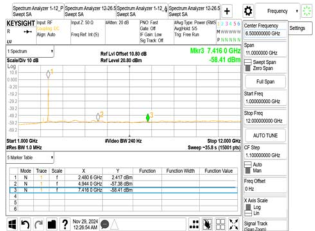
802.11ax_20MHz_2472MHz_RU52_40
