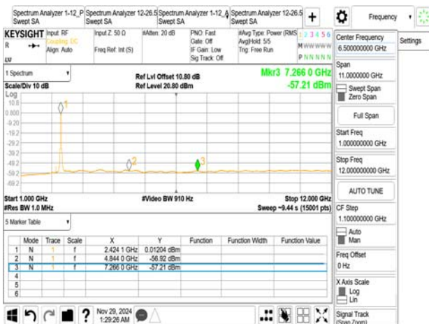
802.11ax_40MHz_2437MHz
