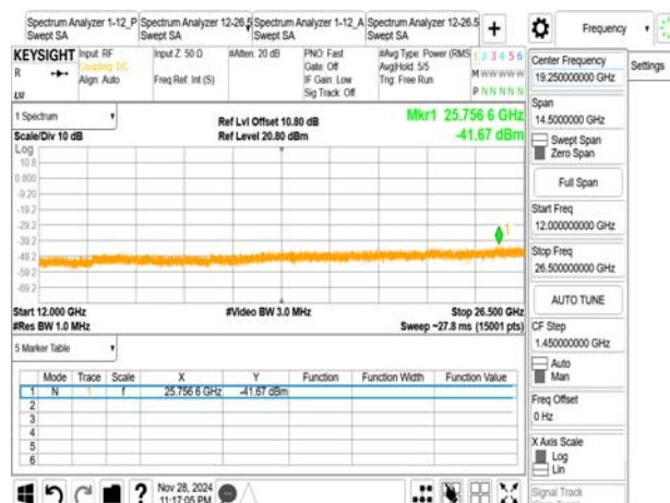
802.11ax_20MHz_2462MHz_RU26_8
