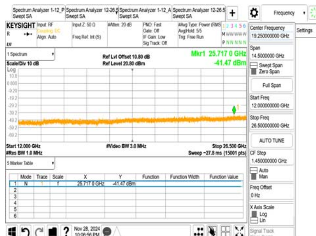
802.11ax_20MHz_2412MHz_RU242
