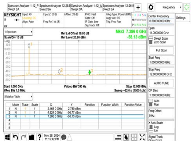
802.11ax_20MHz_2462MHz_RU26_8
