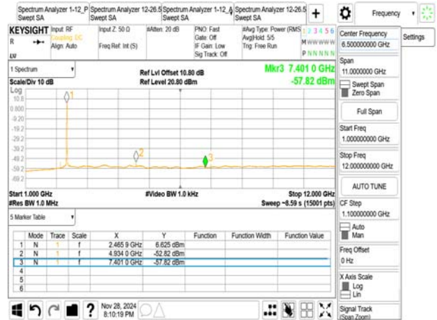
802.11b_20MHz_2472MHz
