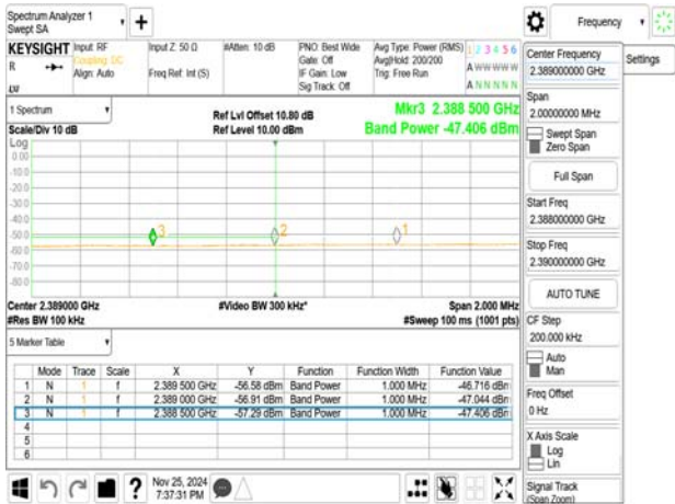
802.11ax_20MHz_2417MHz_RU26_0
