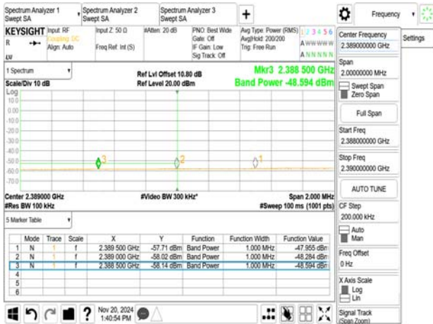
802.11ax_20MHz_2437MHz_R
