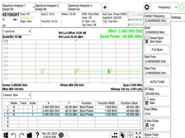
802.11ax_20MHz_2462MHz_RU242
