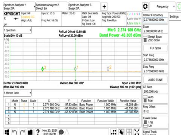
802.11ax_20MHz_2417MHz
