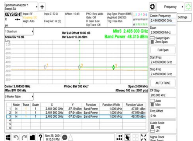
802.11ax_20MHz_2452MHz_RU26_8
