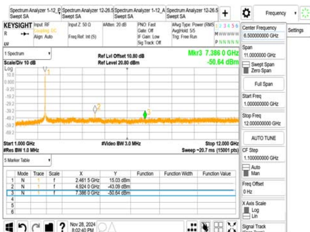
802.11b_20MHz_2462MHz
