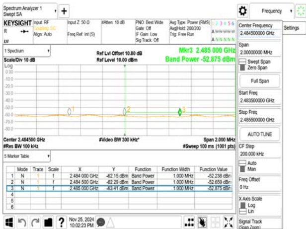
802.11ax_40MHz_2462MHz
