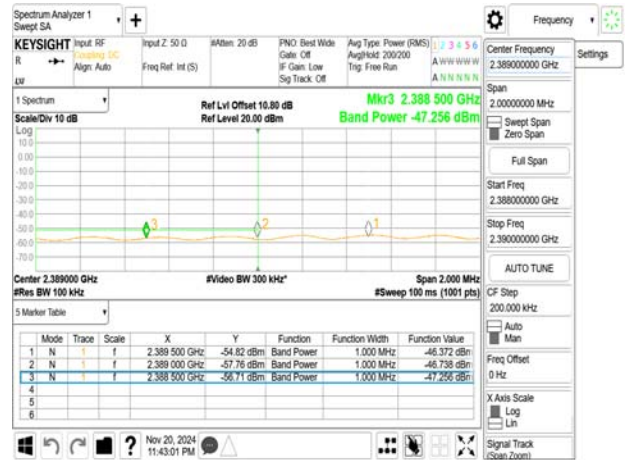
802.11n_40MHz_2432MHz
