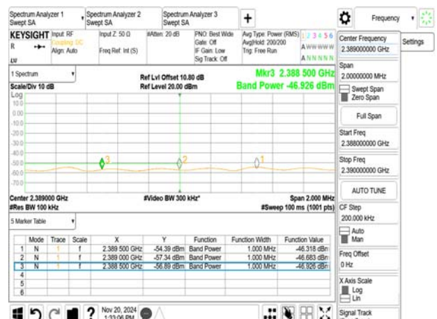
802.11n_40MHz_2437MHz_L
