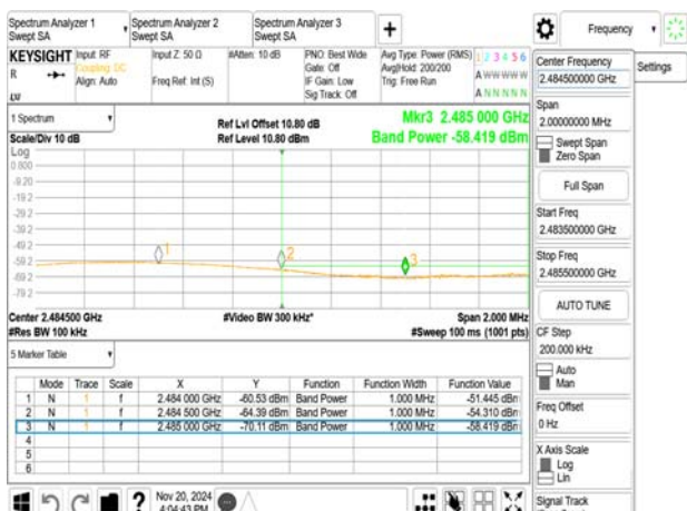
802.11ax_20MHz_2472MHz_RU52_40
