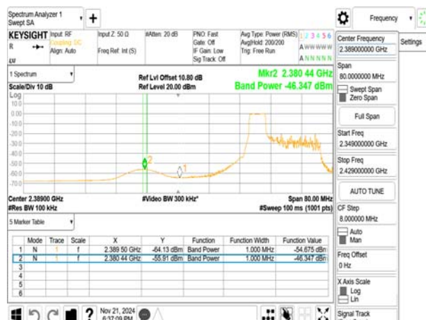
802.11ax_20MHz_2417MHz_RU52_37
