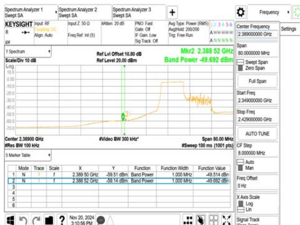
802.11ax_20MHz_2412MHz_RU242
