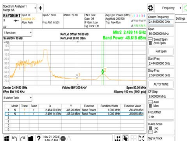
802.11ax_20MHz_2457MHz_RU26_8
