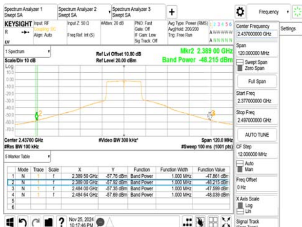
802.11ax_20MHz_2437MHz_RU26_0
