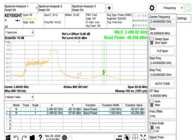
802.11ax_20MHz_2462MHz_RU52_40
