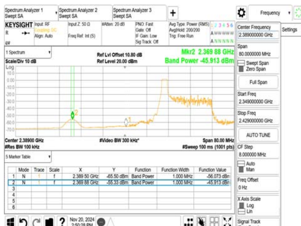
802.11ax_20MHz_2412MHz_RU26_0
