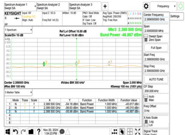
802.11g_20MHz_2417MHz
