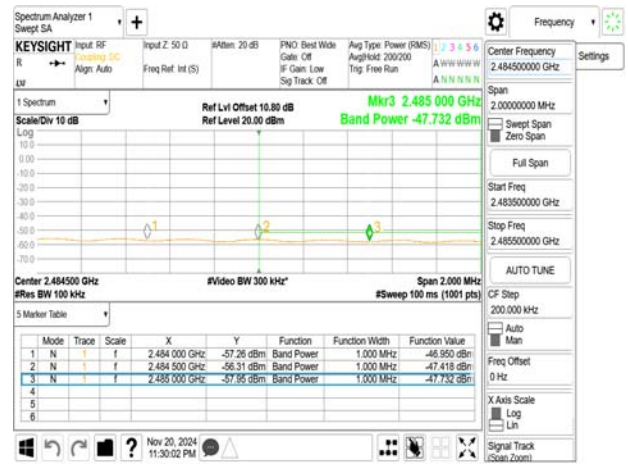
802.11n_20MHz_2457MHz
