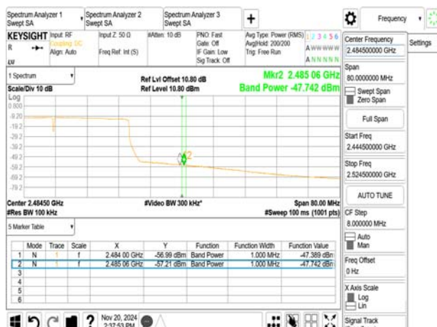
802.11ax_40MHz_2452MHz
