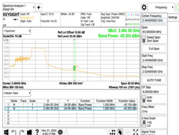
802.11ax_20MHz_2457MHz_RU242
