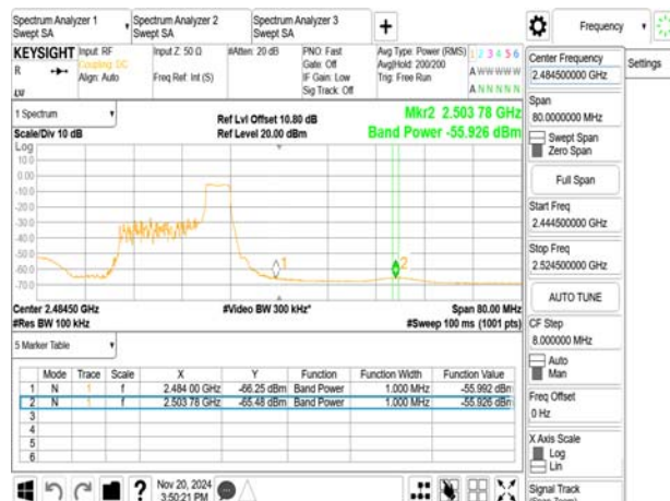
802.11ax_20MHz_2472MHz
