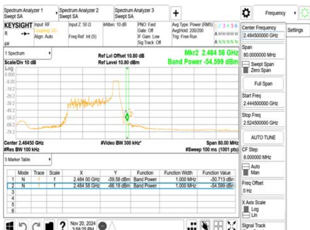
802.11ax_20MHz_2472MHz_RU26_8
