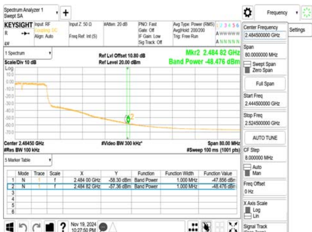
802.11n_20MHz_2452MHz
