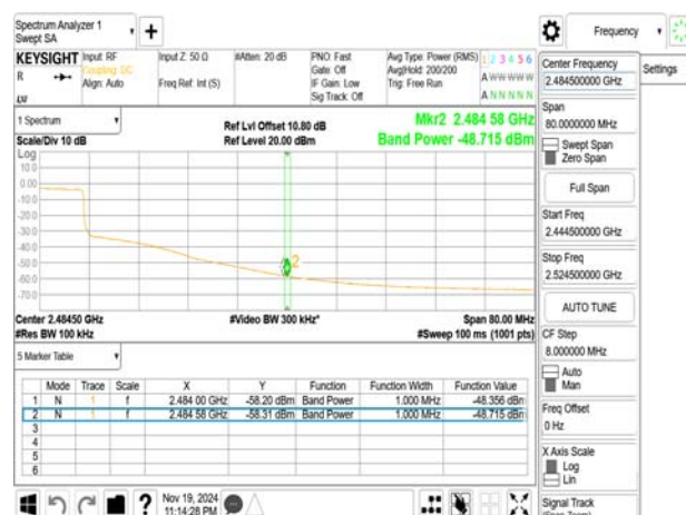
802.11ax_20MHz_2442MHz
