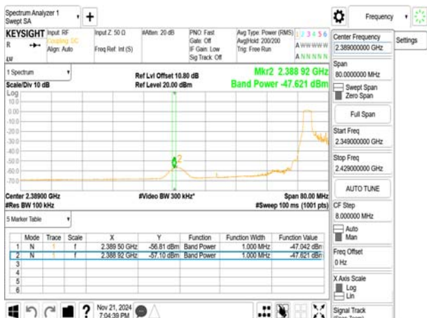
802.11ax_20MHz_2432MHz_RU52_37
