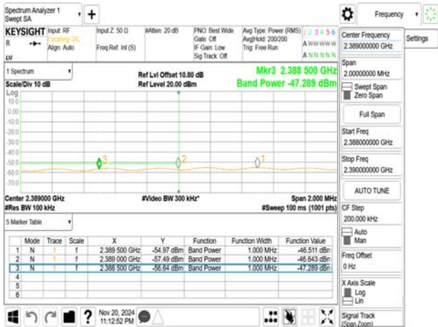
802.11g_20MHz_2427MHz
