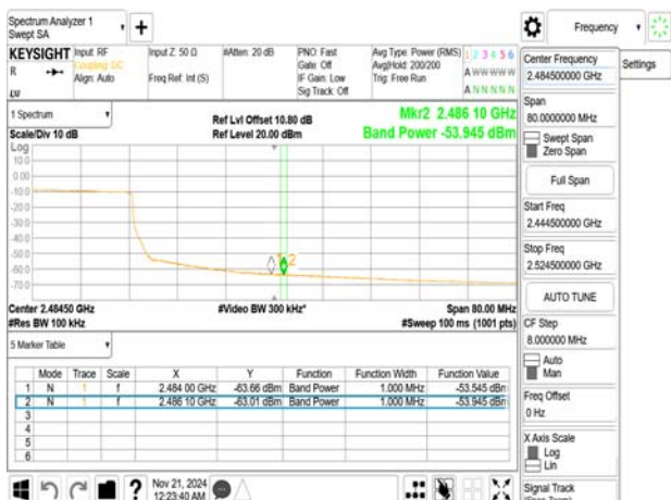
802.11ax_40MHz_2442MHz_RU484
