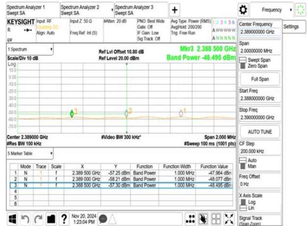
802.11g_20MHz_2437MHz_R
