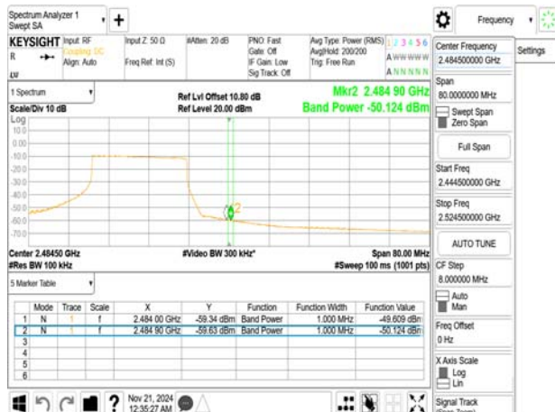
802.11ax_40MHz_2457MHz_RU484
