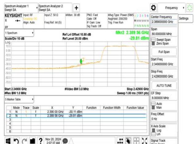
802.11n_20MHz_2412MHz
