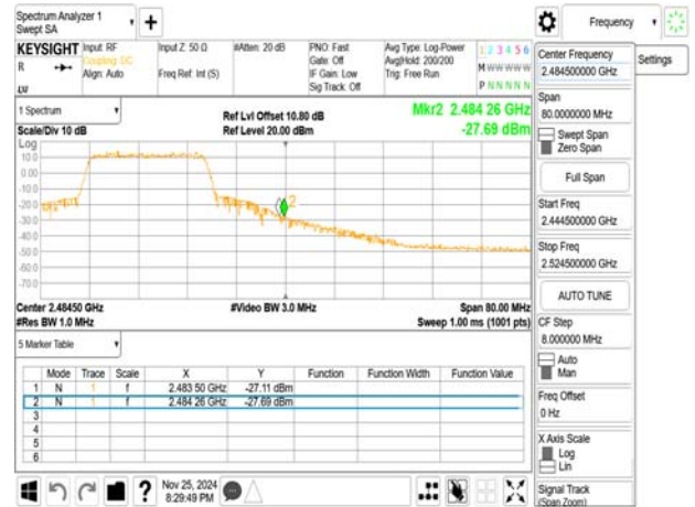
802.11ax_20MHz_2462MHz_RU26_8
