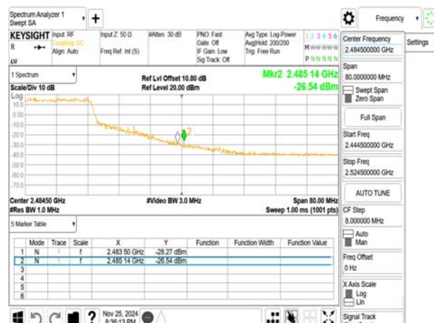
802.11ax_20MHz_2452MHz_RU242
