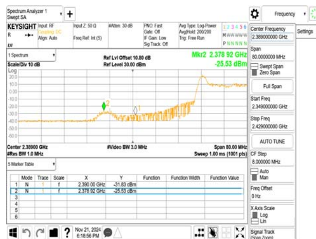
802.11ax_20MHz_2422MHz_RU52_37
