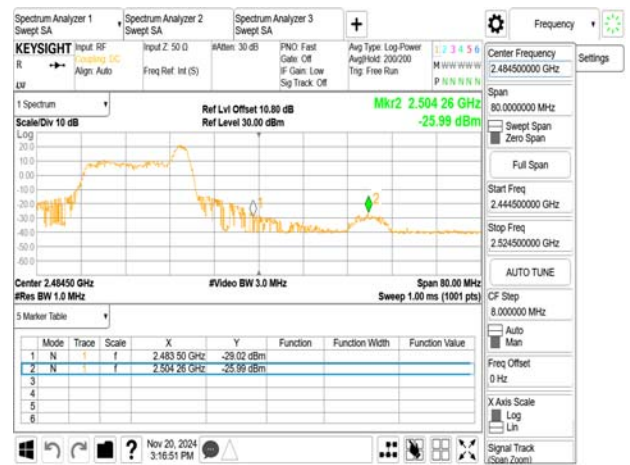
802.11ax_20MHz_2462MHz_RU52_40
