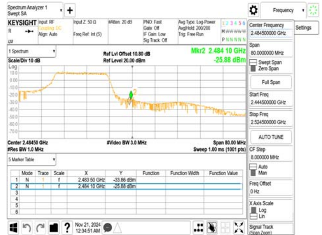
802.11ax_40MHz_2457MHz_RU484
