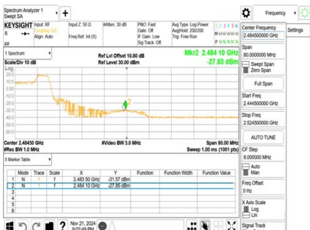
802.11ax_20MHz_2447MHz_RU52_40
