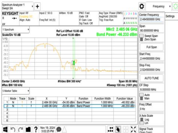
802.11b_20MHz_2467MHz
