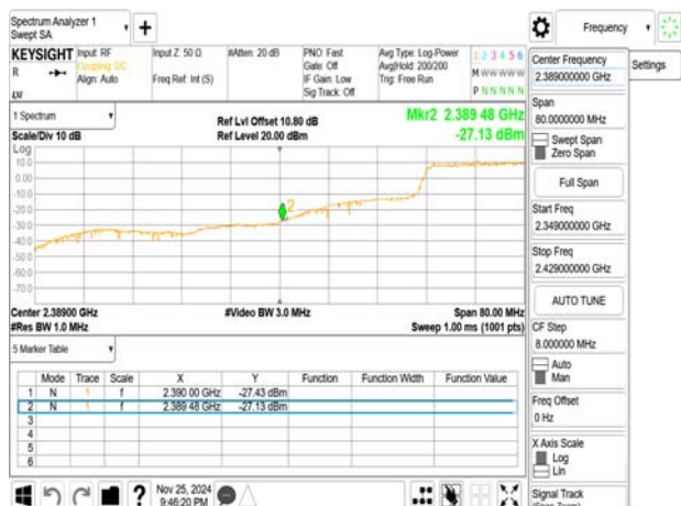
802.11ax_40MHz_2437MHz
