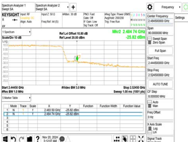
802.11ax_40MHz_2457MHz
