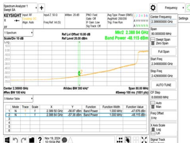
802.11n_20MHz_2437MHz
