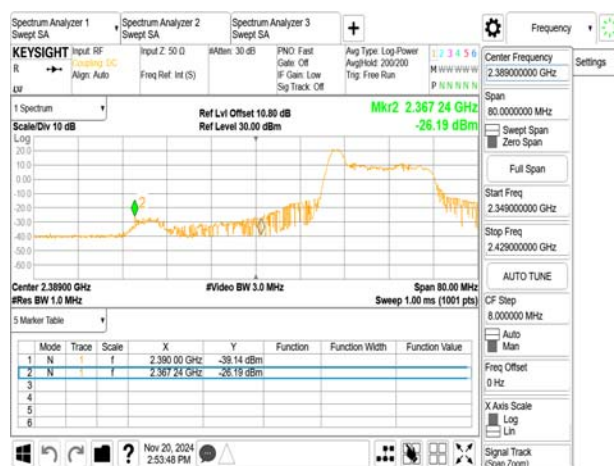
802.11ax_20MHz_2412MHz_RU26_0
