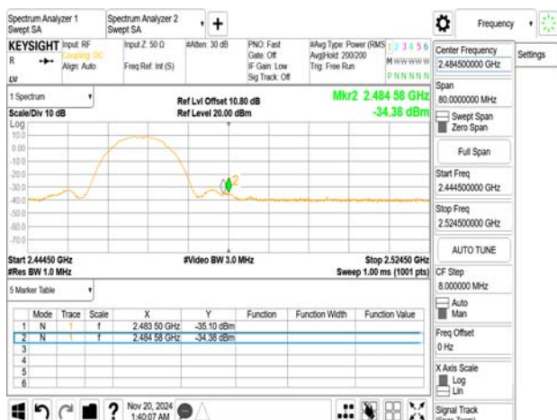
802.11b_20MHz_2467MHz
