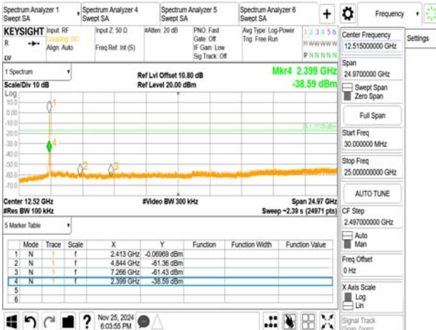
802.11ax_40MHz_Chain0_2422MHz_RU484
