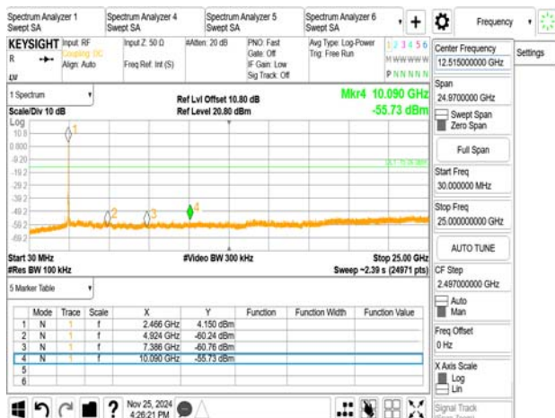
802.11ax_20MHz_Chain0_2462MHz_RU242
