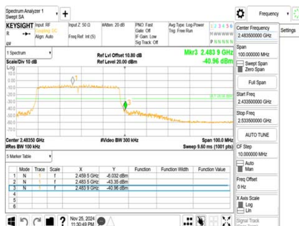
802.11ax_40MHz_Chain0_2462MHz_RU484
