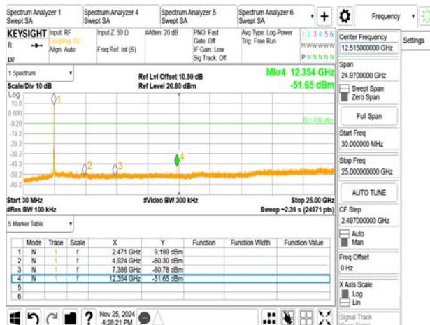
802.11ax_20MHz_Chain0_2462MHz_RU52_40
