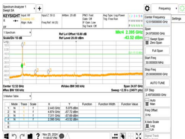
802.11ax_20MHz_Chain0_2437MHz_RU242
