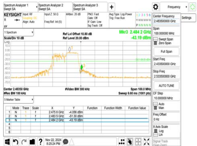
802.11ax_20MHz_Chain0_2472MHz_RU26_8
