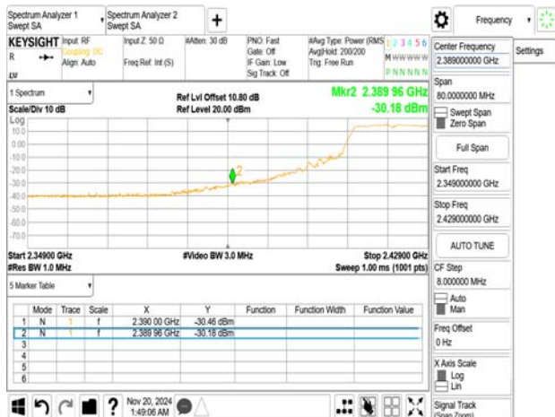
802.11g_20MHz_2427MHz
