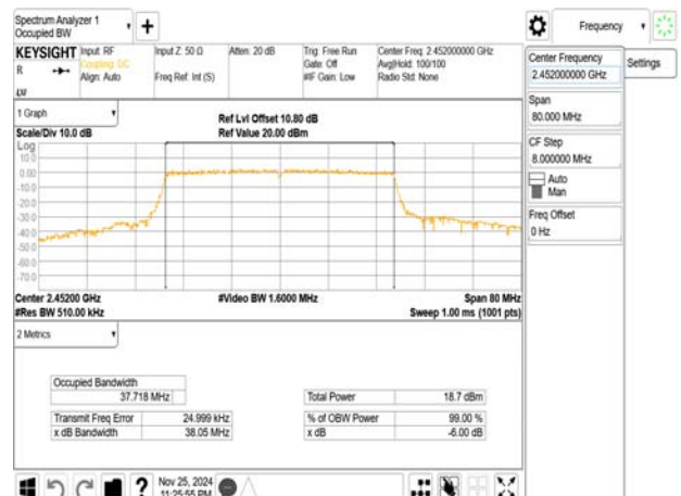
802.11ax_40MHz_Chain0_2452MHz_RU484
