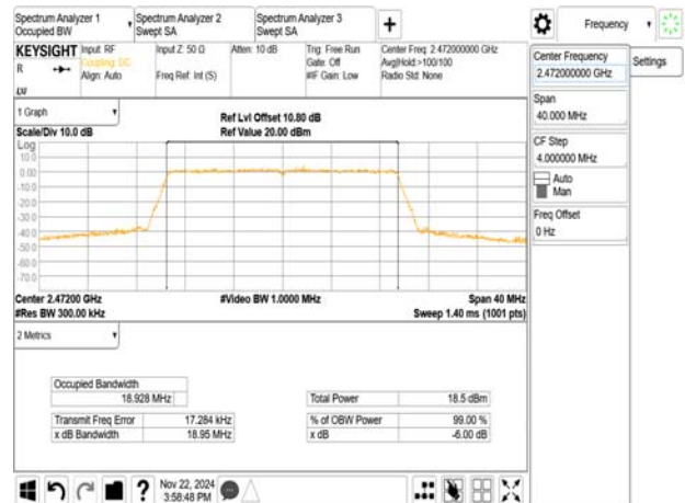
802.11ax_20MHz_Chain0_2472MHz_RU242
