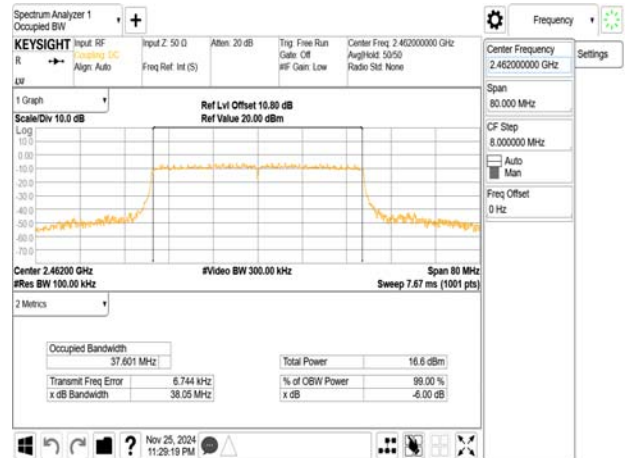
802.11ax_40MHz_Chain0_2462MHz_RU484
