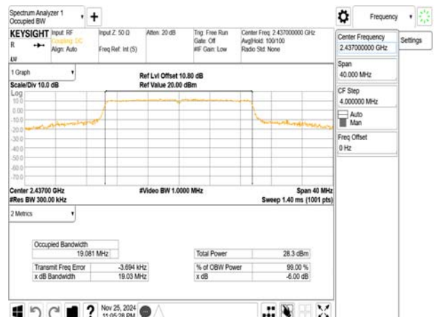
802.11ax_20MHz_Chain0_2437MHz_RU242
