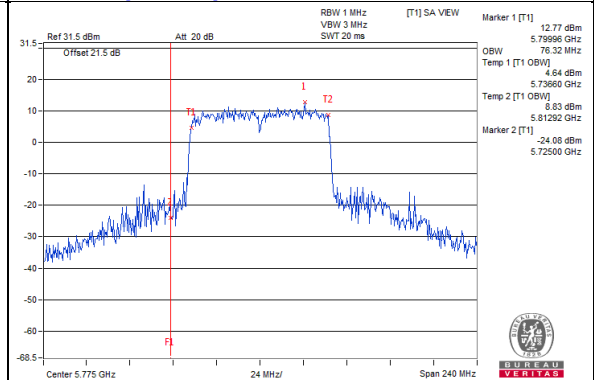
802.11ac(VHT80)_Chain3 / CH155
