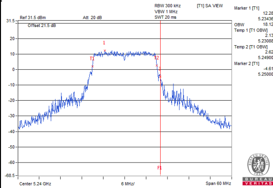
802.11ac(VHT20)_Chain2 / CH48
