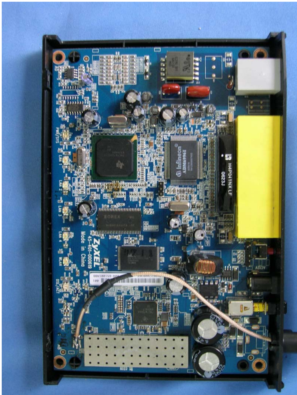
(5) EUT Photo
