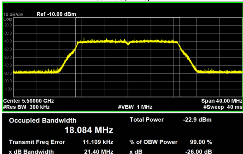
802.11ac (VHT20)
