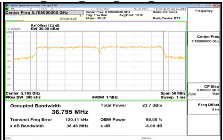
IC 802.11n 40MHz Chain1 5795MHz
