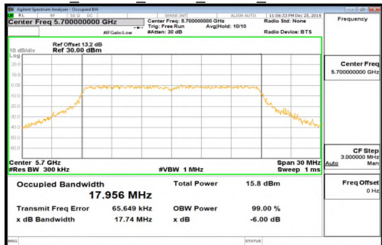
IC 802.11n 20MHz Chain0 5700MHz
