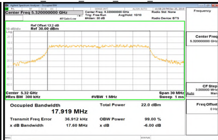
IC 802.11n 20MHz Chain1 5320MHz
