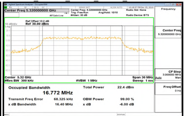
IC 802.11a 20MHz Chain1 5320MHz
