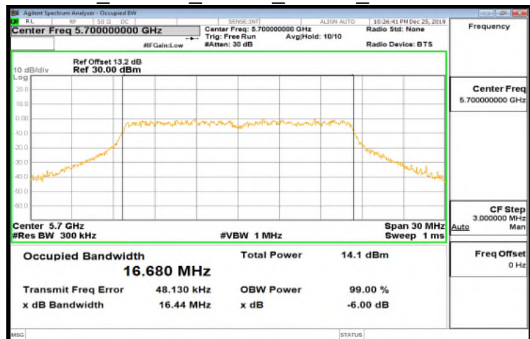
IC 802.11a 20MHz Chain1 5700MHz
