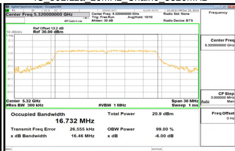
IC 802.11a 20MHz Chain0 5320MHz
