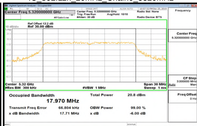
IC 802.11n 20MHz Chain0 5320MHz
