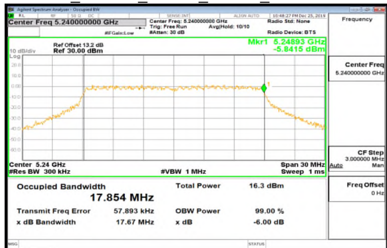
IC 802.11n 20MHz Chain1 5240MHz
