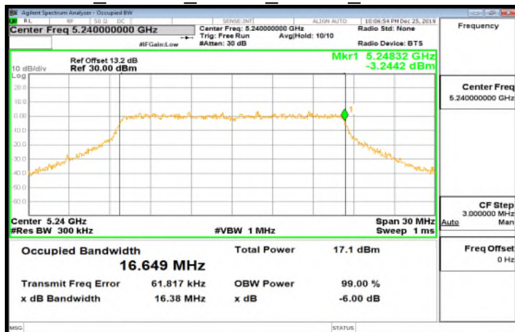
IC 802.11a 20MHz Chain1 5240MHz
