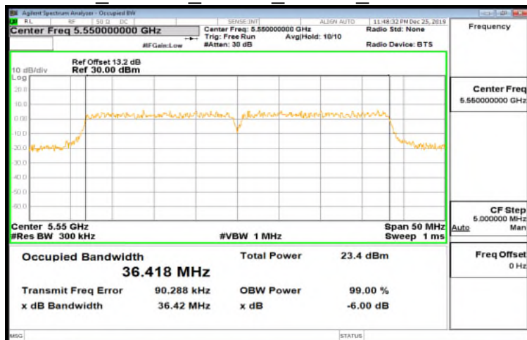
IC 802.11n 40MHz Chain1 5550MHz
