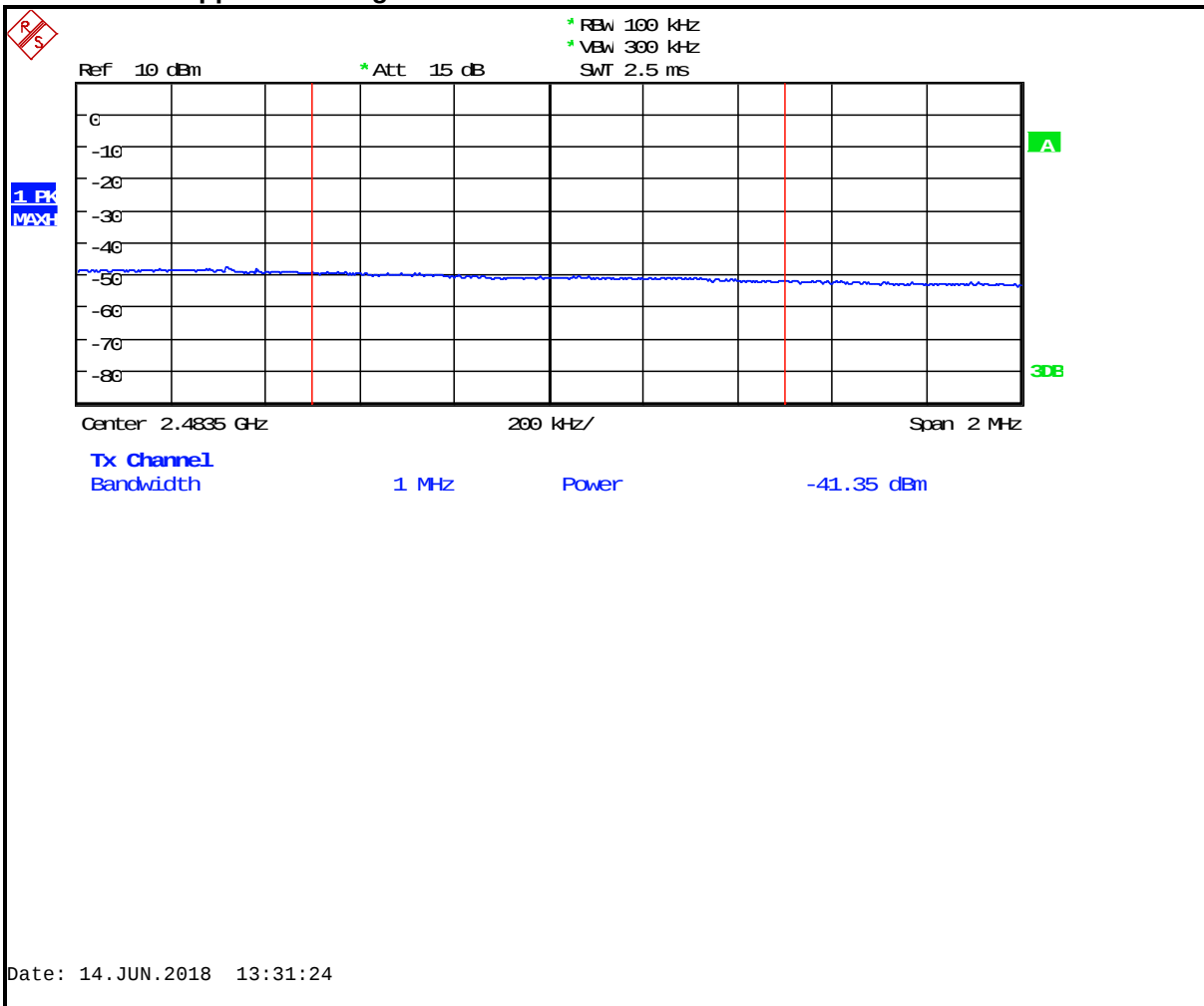
Plot 4-10: Upper Band Edge Peak: BLE
