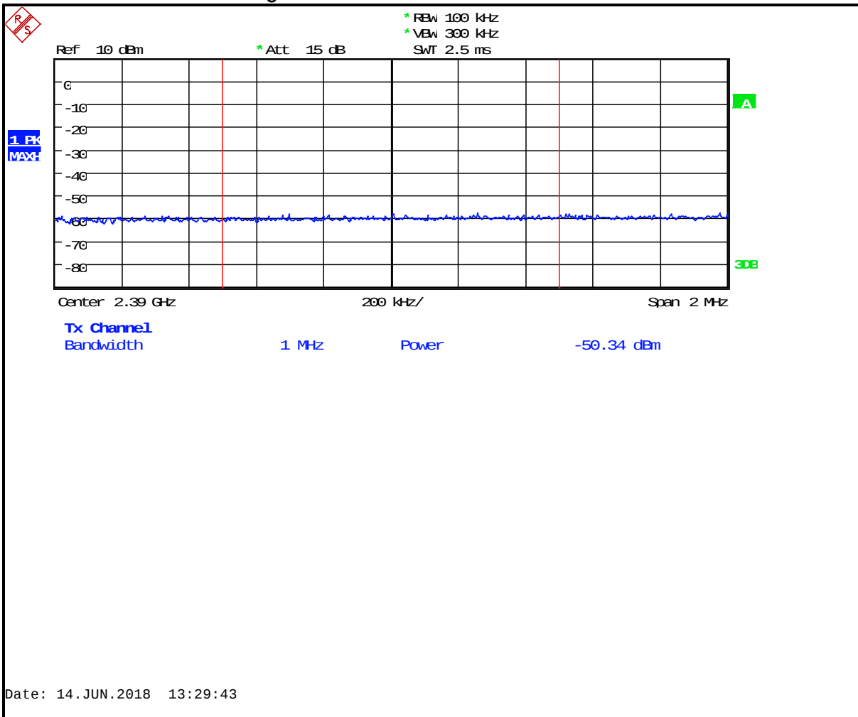
Plot 4-2: Lower Band Edge Peak: BLE
