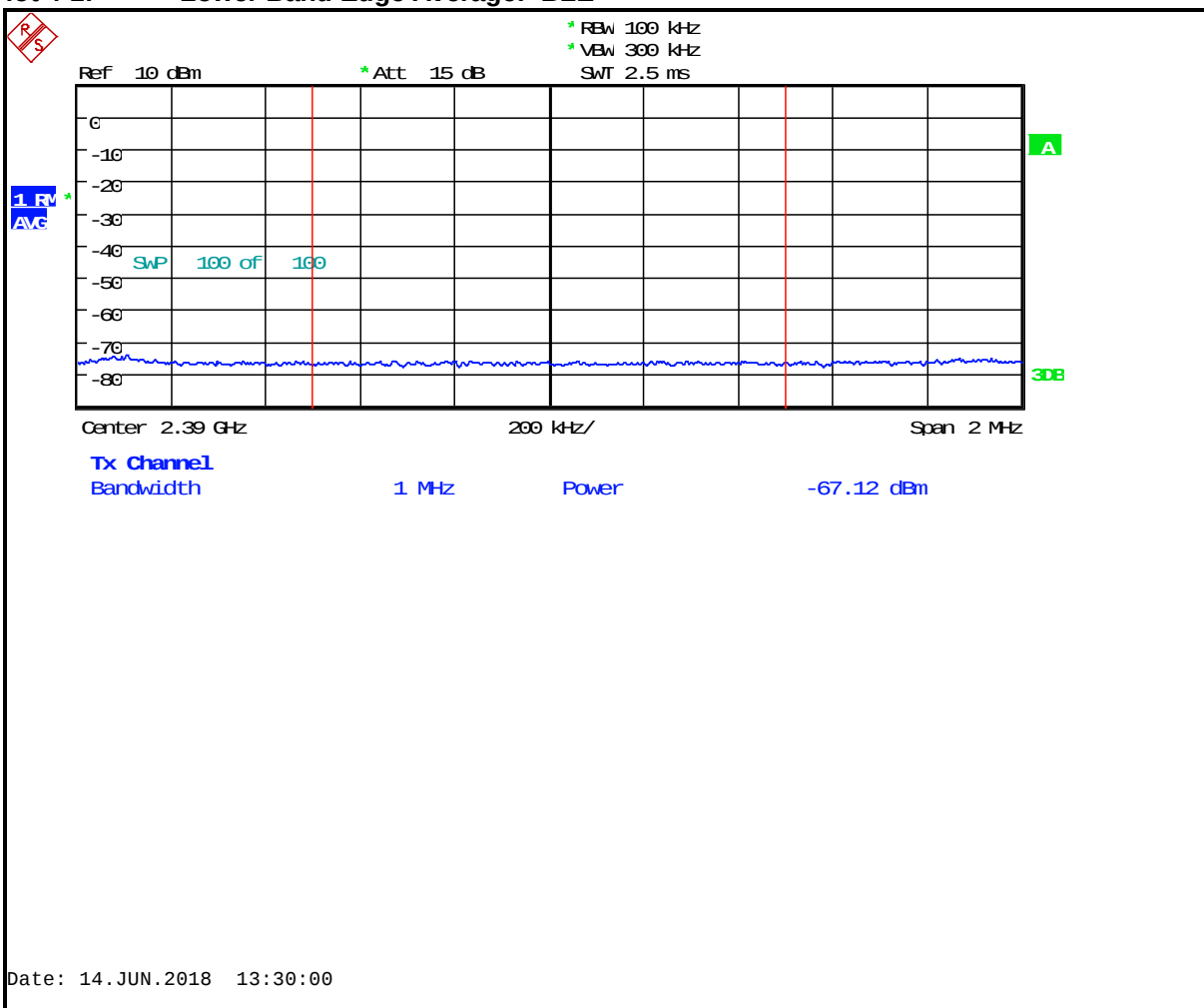
Plot 4-1: Lower Band Edge Average: BLE
