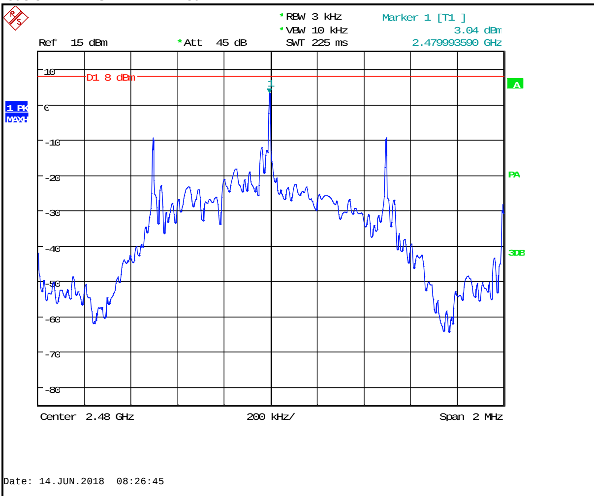
Plot 8-3: PSD - BLE - 2480 MHz
