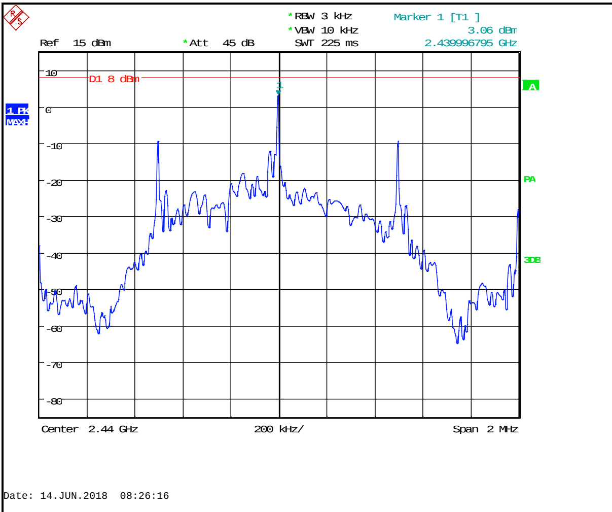
Plot 8-2: PSD - BLE - 2440 MHz
