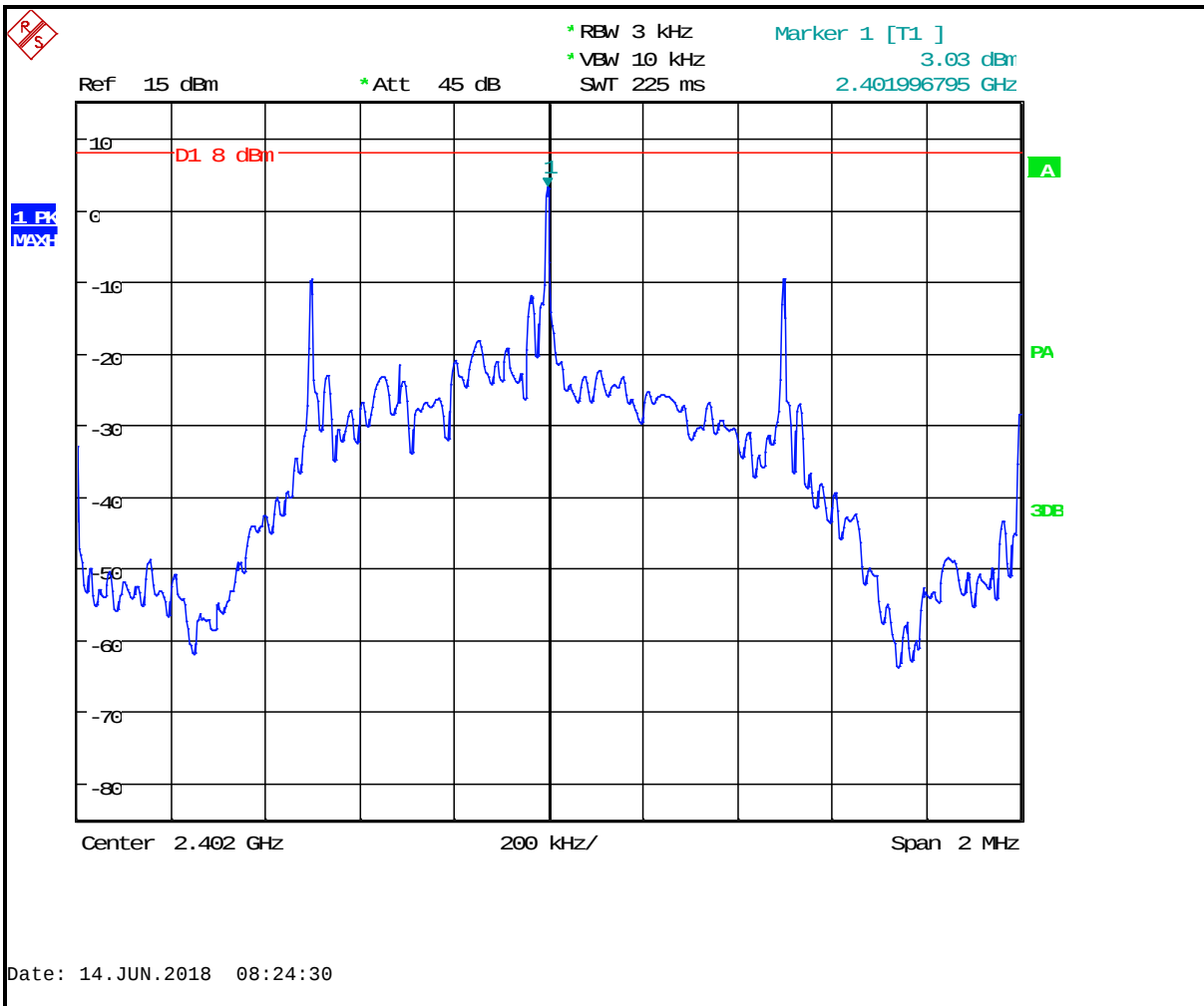
Plot 8-1: PSD - BLE - 2402 MHz
