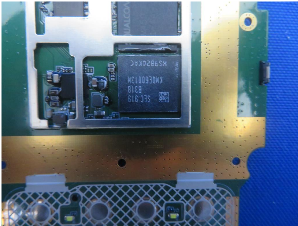
(15) EUT Photo
