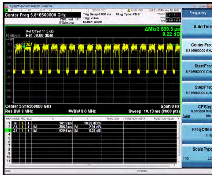
11AX20MIMO_Ant2_5825_26Tone_RU4
