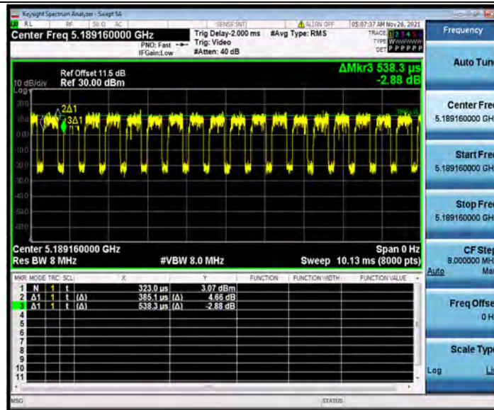
11AX40MIMO_Ant1_5190_26Tone_RU17
