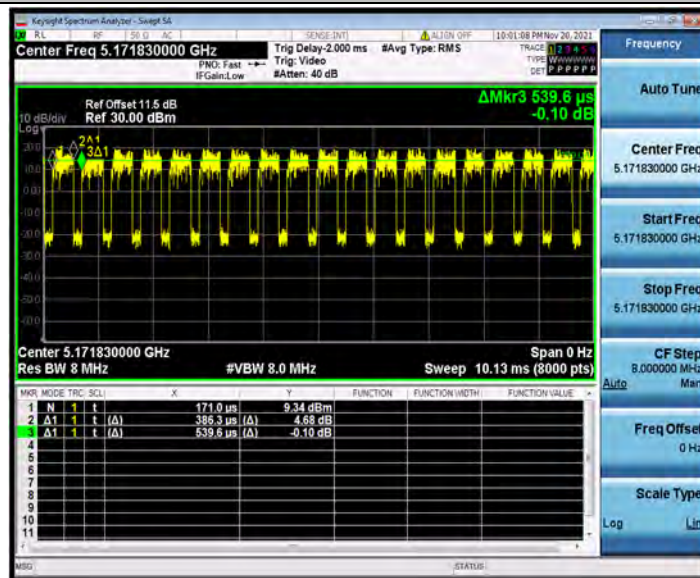
11AX40MIMO_Ant1_5190_26Tone_RU8
