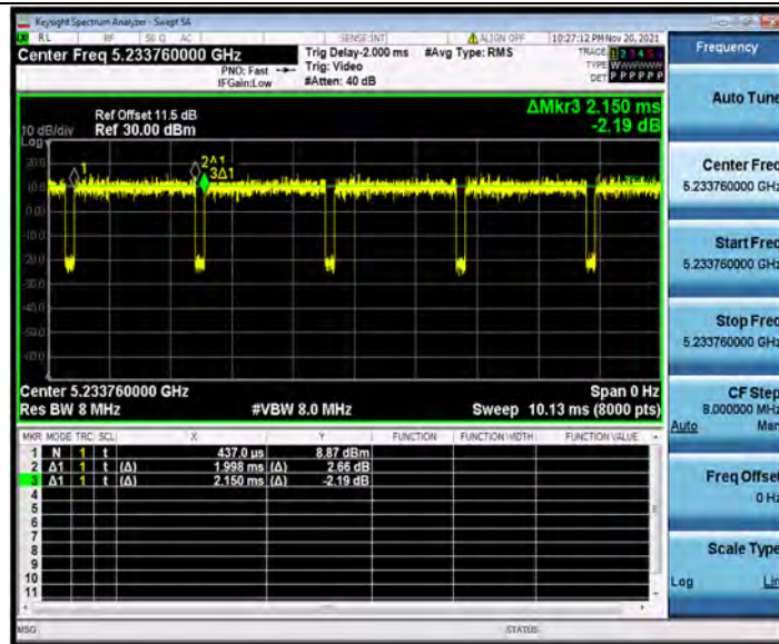
11AX40MIMO_Ant2_5230_26Tone_RU0
