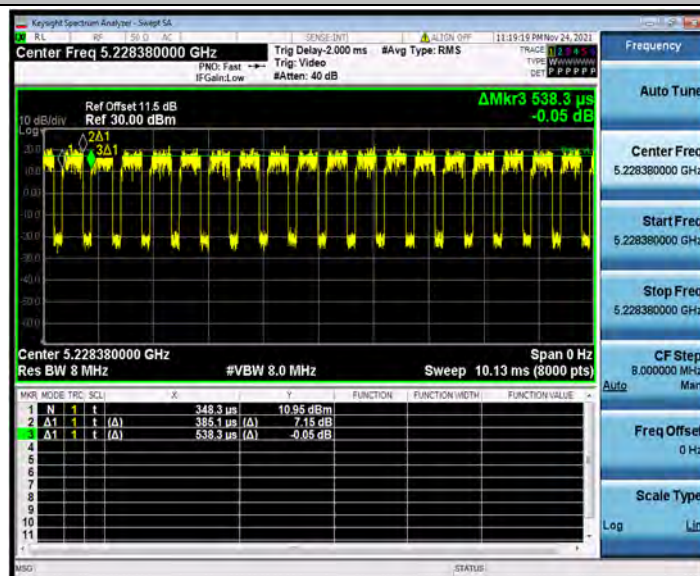
11AX40MIMO_Ant2_5230_26Tone_RU8
