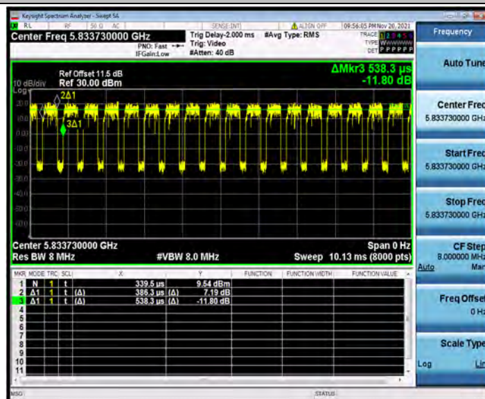
11AX20MIMO_Ant2_5825_26Tone_RU8
