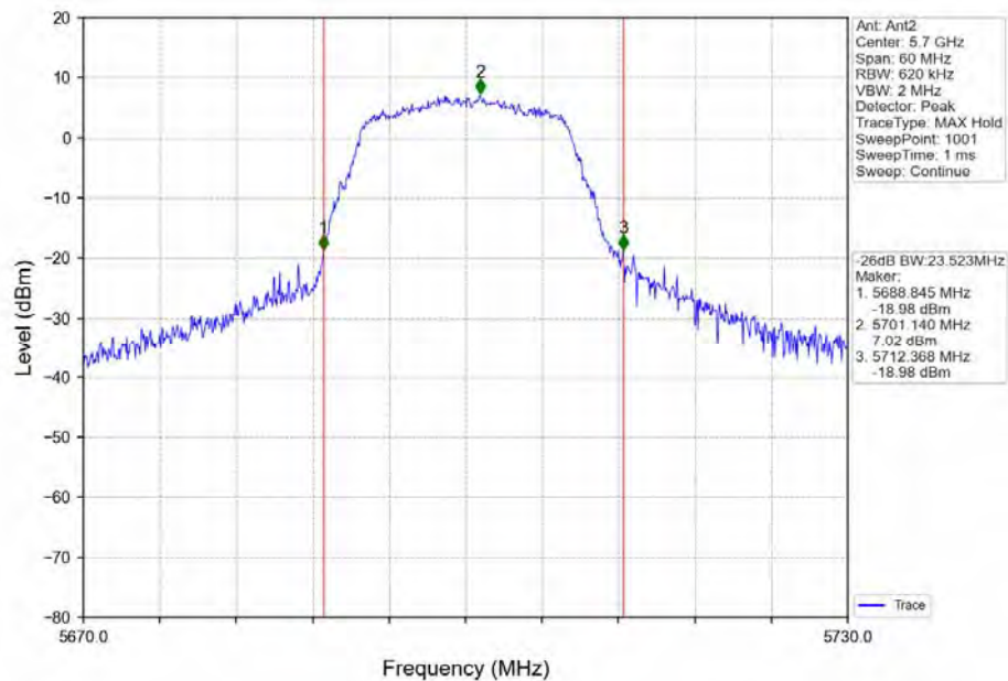
802.11a_HCH_5700MHz_Ant2_NTNV
