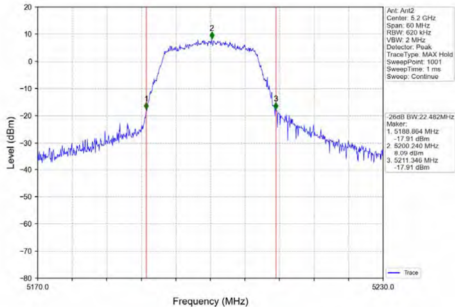
802.11a_MCH_5200MHz_Ant2_NTNV
