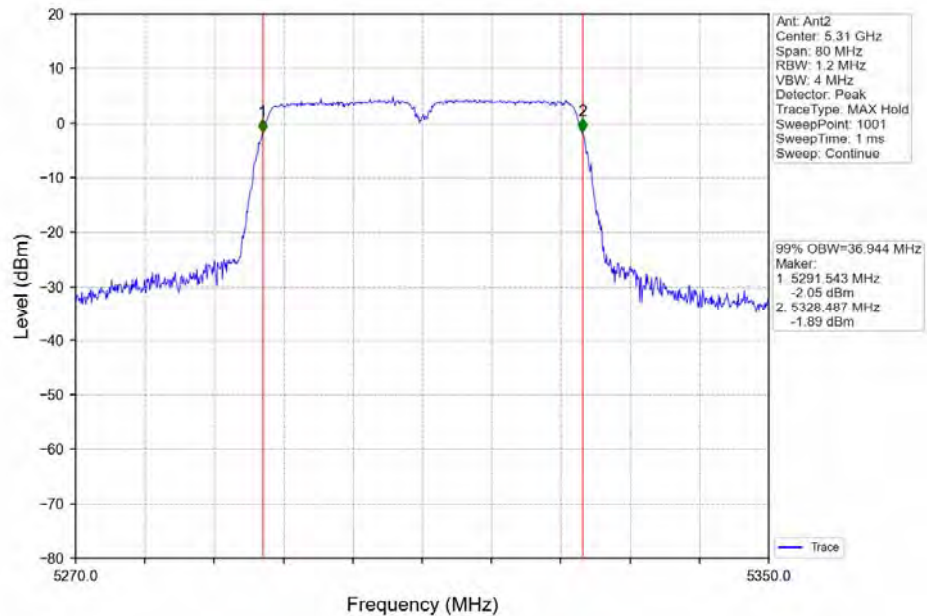
802.11ac(VHT40) HCH_5310MHz_Ant2_NTNV
