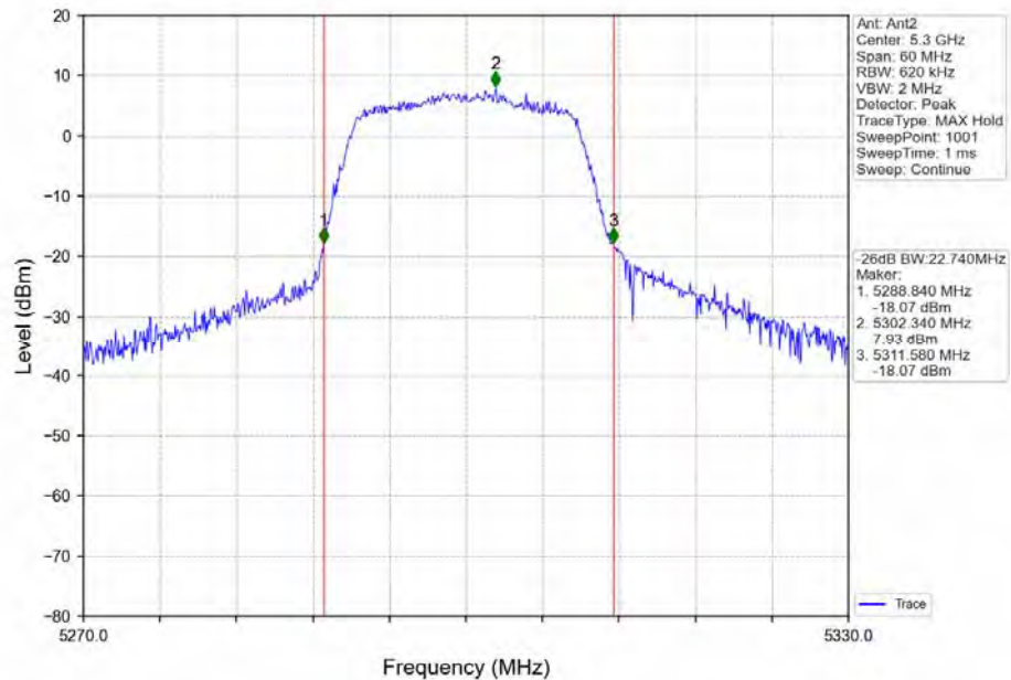
802.11n(HT20) MCH_5300MHz_Ant2_NTNV
