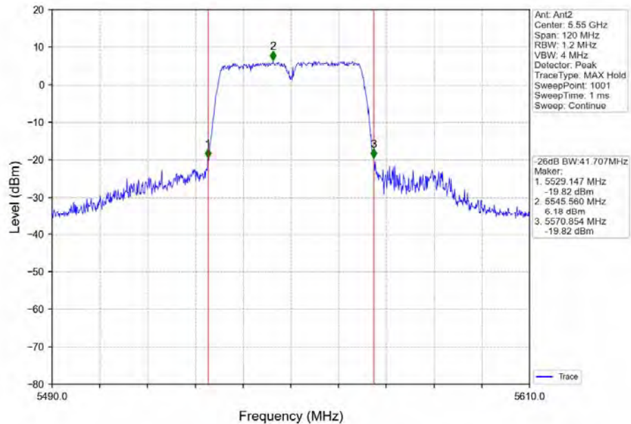
802.11n(HT40) MCH_5550MHz_Ant2_NTNV
