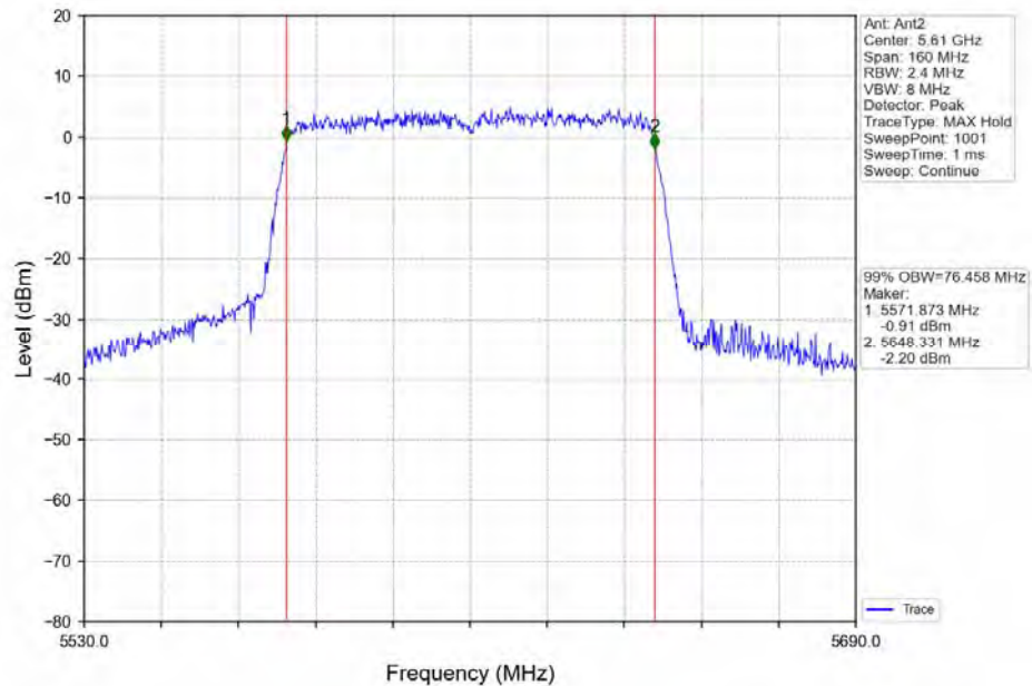
802.11ac(VHT80) HCH_5610MHz_Ant2_NTNV
