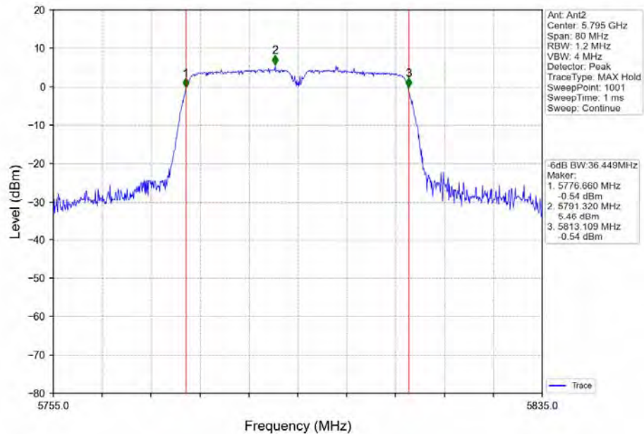
802.11ac(VHT40) HCH_5795MHz_Ant2_NTNV
