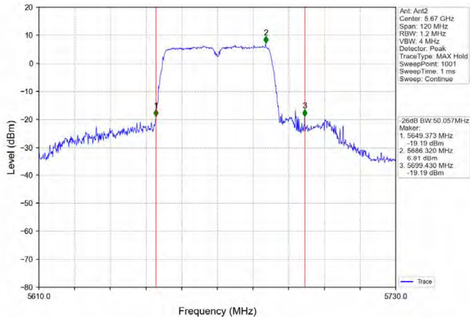
802.11n(HT40) HCH 5670MHz Ant2_NTNV
