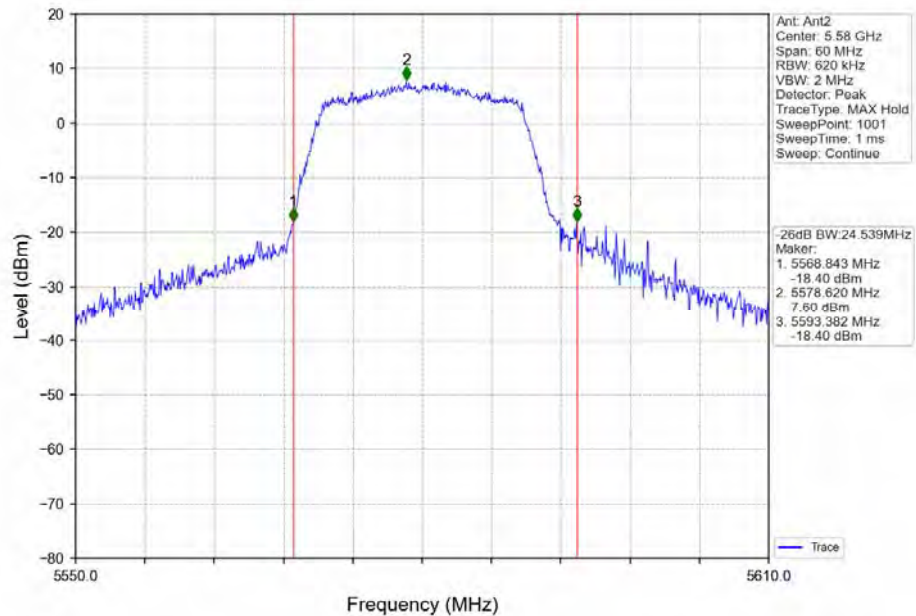
802.11n(HT20) MCH_5580MHz_Ant2_NTNV
