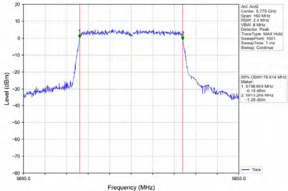
802.11ac(VHT80) MCH_5775MHz_Ant2_NTNV
