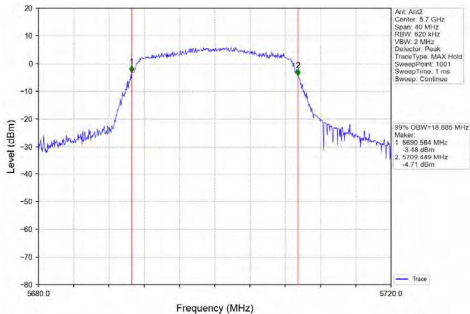
802.11ac(VHT20) HCH_5700MHz_Ant2_NTNV
