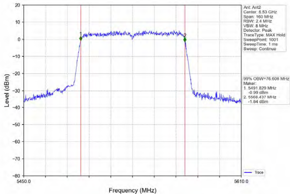
802.11ac(VHT80)_LCH_5530MHz_Ant2_NTNV
