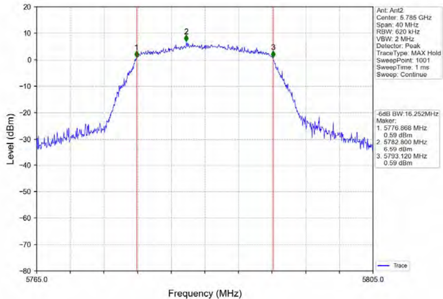
802.11a_MCH_5785MHz_Ant2_NTNV
