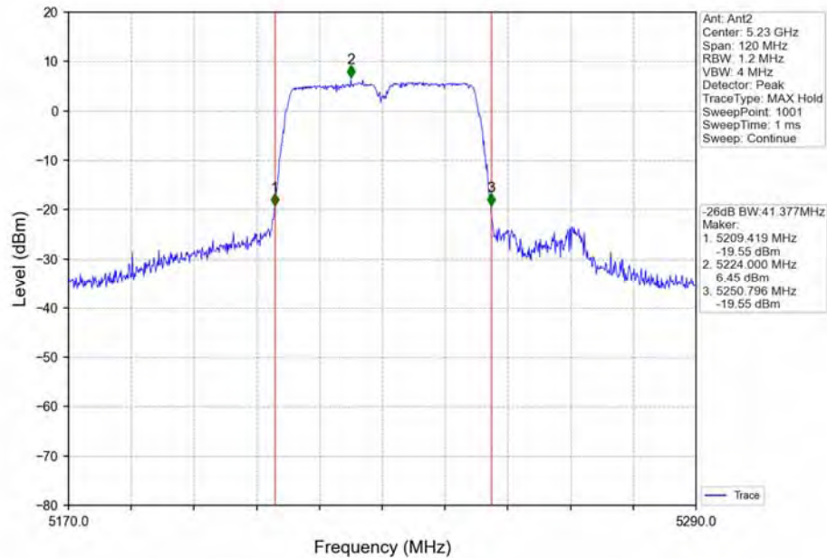
802.11n(HT40)_HCH_5230MHz_Ant2_NTNV
