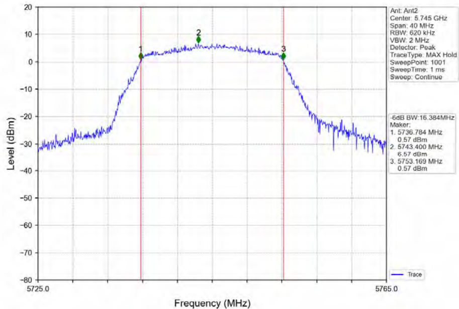
802.11a_LCH_5745MHz_Ant2_NTNV
