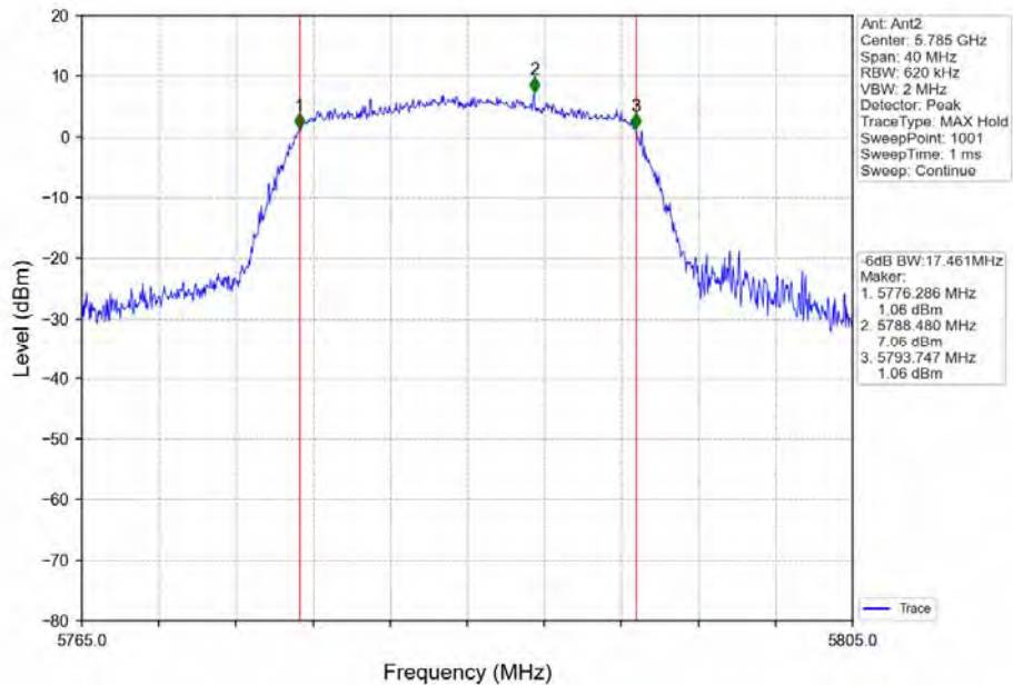
802.11n(HT20) MCH_5785MHz_Ant2_NTNV
