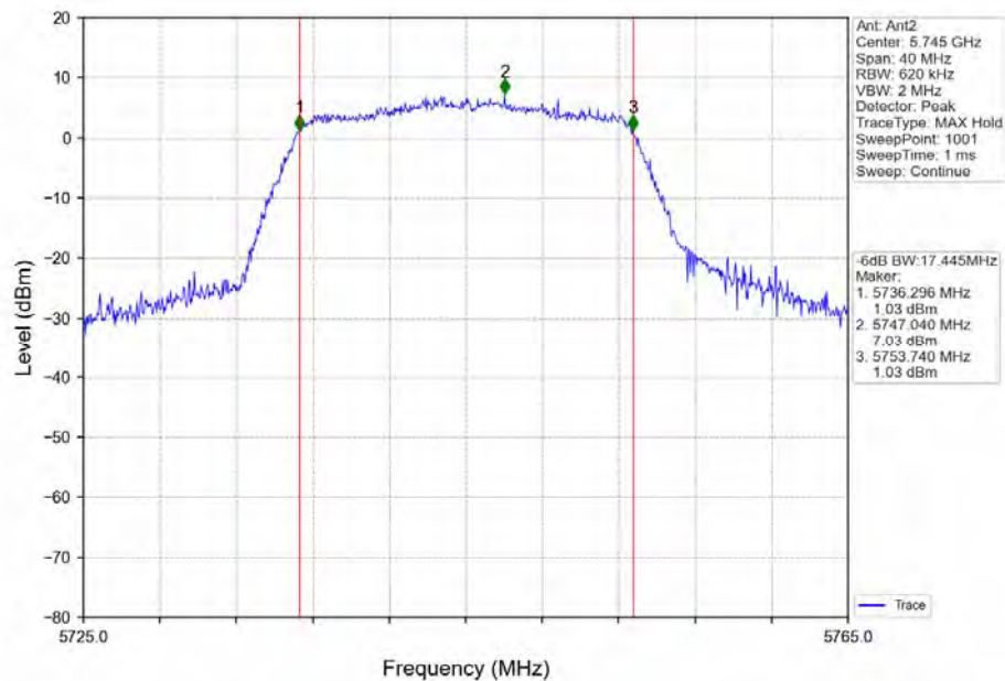
802.11n(HT20) LCH_5745MHz_Ant2_NTNV
