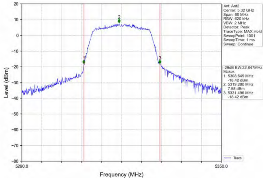
802.11n(HT20)_HCH_5320MHz_Ant2_NTNV
