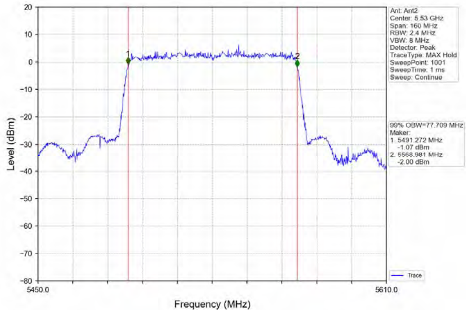
802.11ax(HEW80)_LCH_5530MHz_Ant2_NTNV
