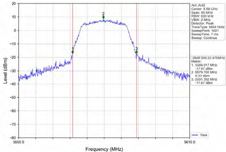
802.11a_MCH_5580MHz_Ant2_NTNV
