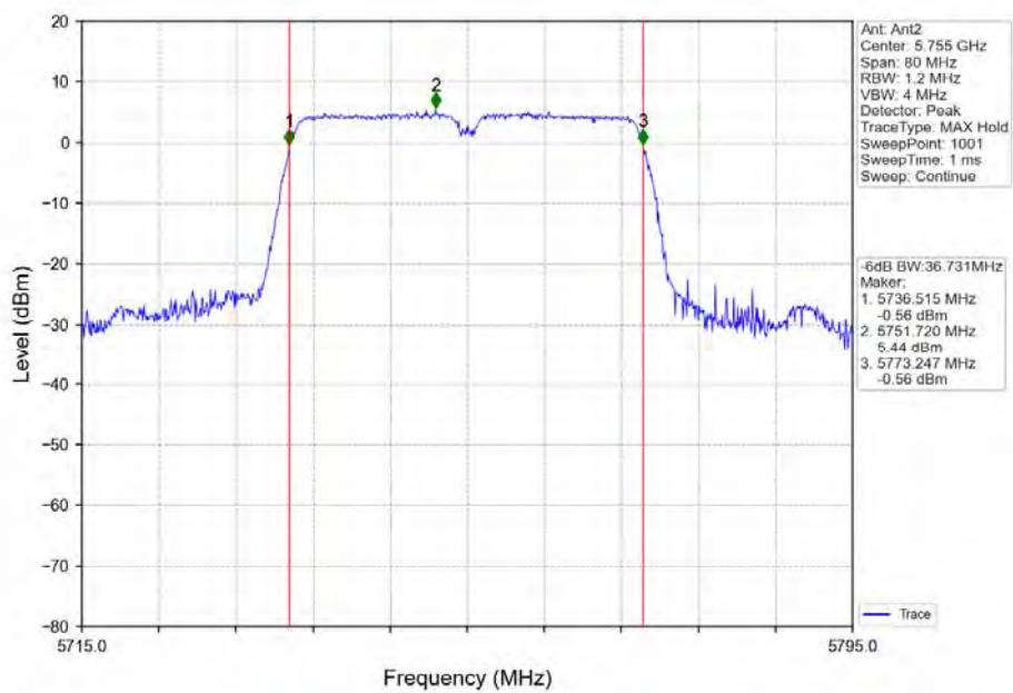
802.11ac(VHT40) LCH_5755MHz_Ant2_NTNV
