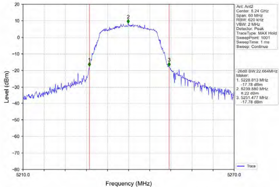
802.11a_HCH_5240MHz_Ant2_NTNV
