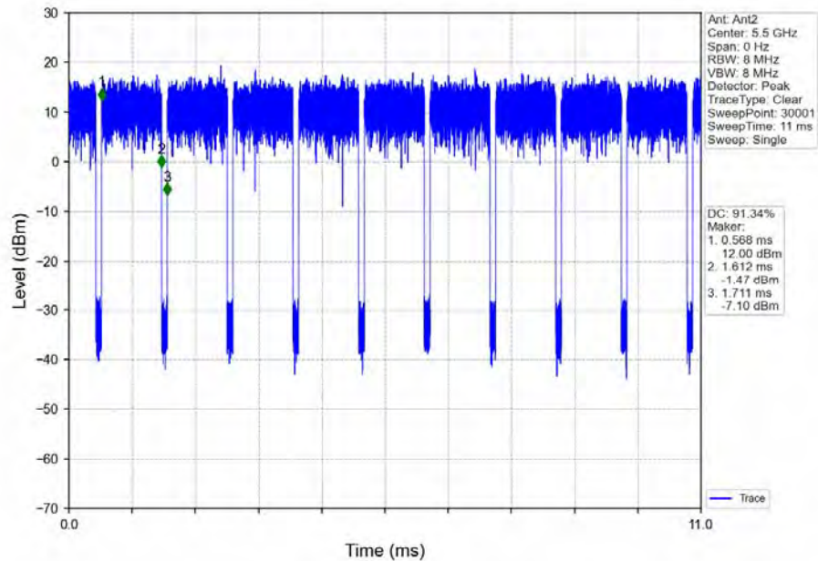
802.11ax(HEW20)_LCH_5500MHz_Ant2_NTNV
