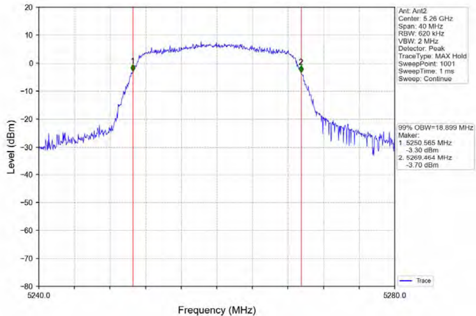
802.11n(HT20) LCH_5260MHz_Ant2_NTNV
