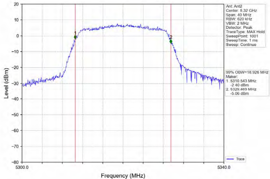
802.11n(HT20)_HCH_5320MHz_Ant2_NTNV
