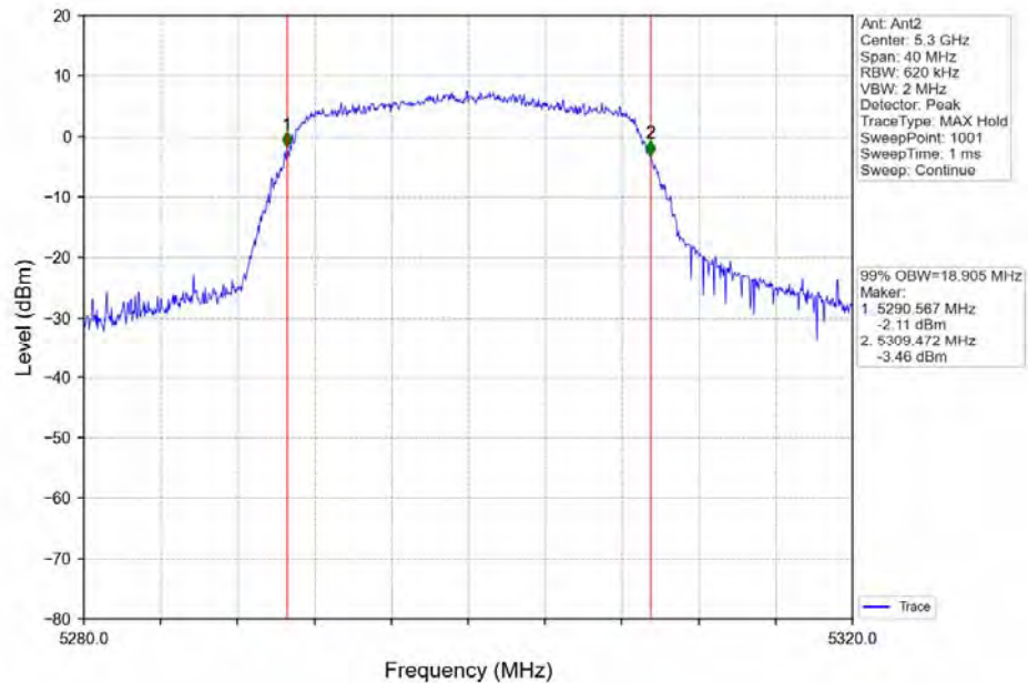
802.11n(HT20) MCH_5300MHz_Ant2_NTNV
