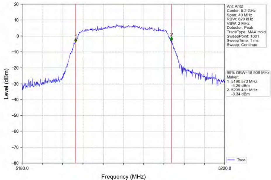
802.11n(HT20) MCH_5200MHz_Ant2_NTNV
