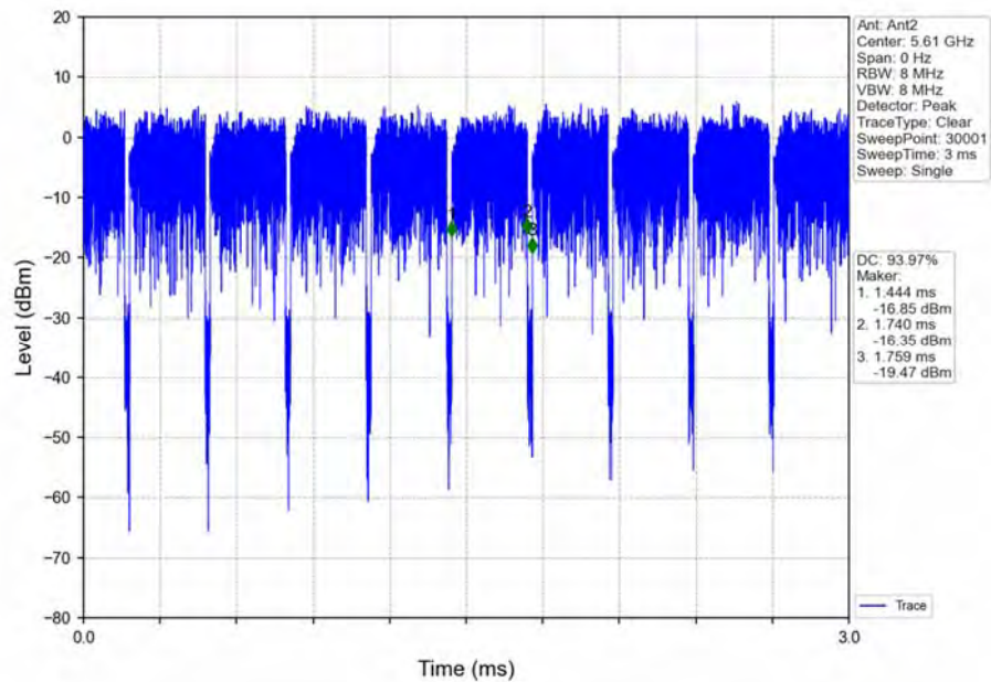
802.11ax(HEW80)_HCH_5610MHz_Ant2_NTNV
