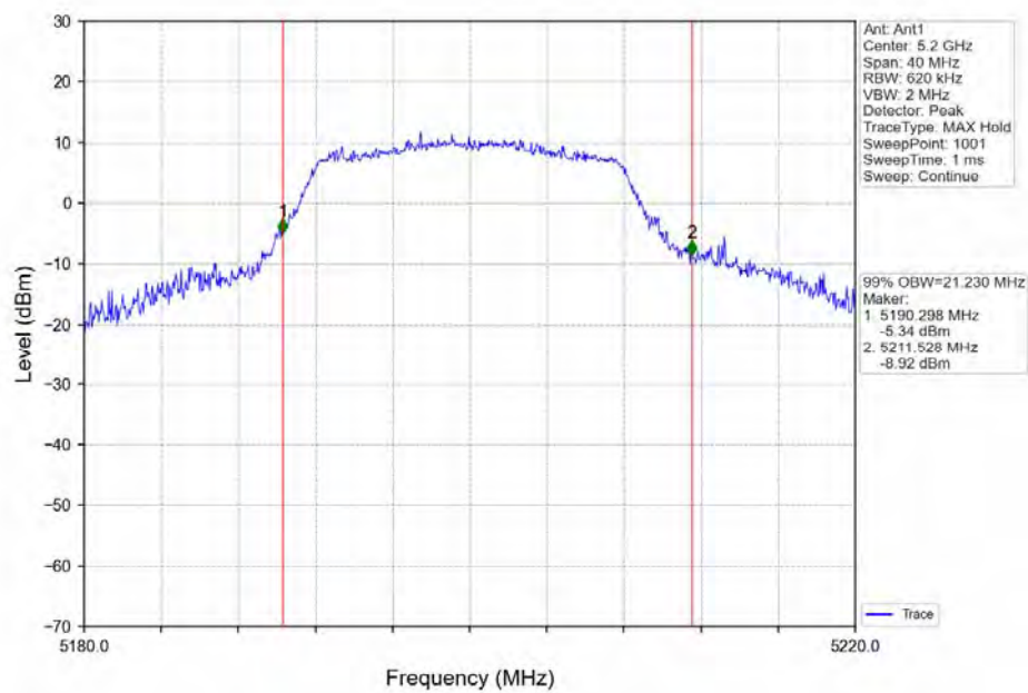
802.11a_MCH_5200MHz_Ant1_NTNV
