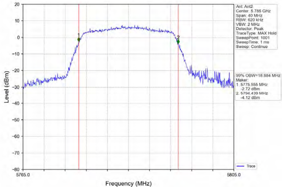
802.11n(HT20) MCH_5785MHz_Ant2_NTNV
