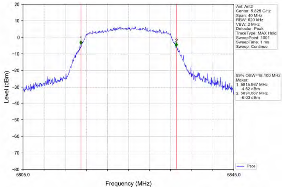
802.11a_HCH_5825MHz_Ant2_NTNV
