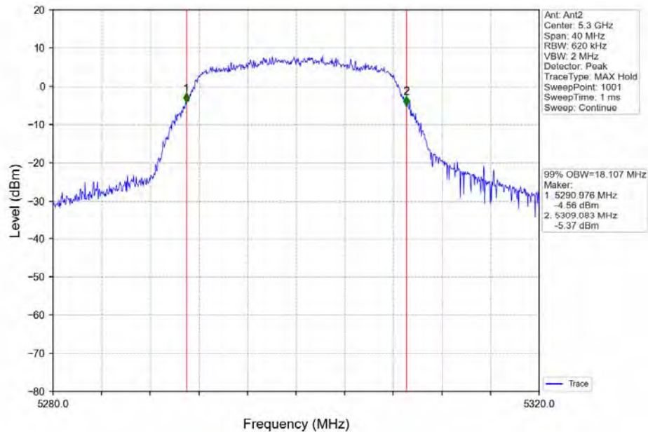
802.11a_MCH_5300MHz_Ant2_NTNV
