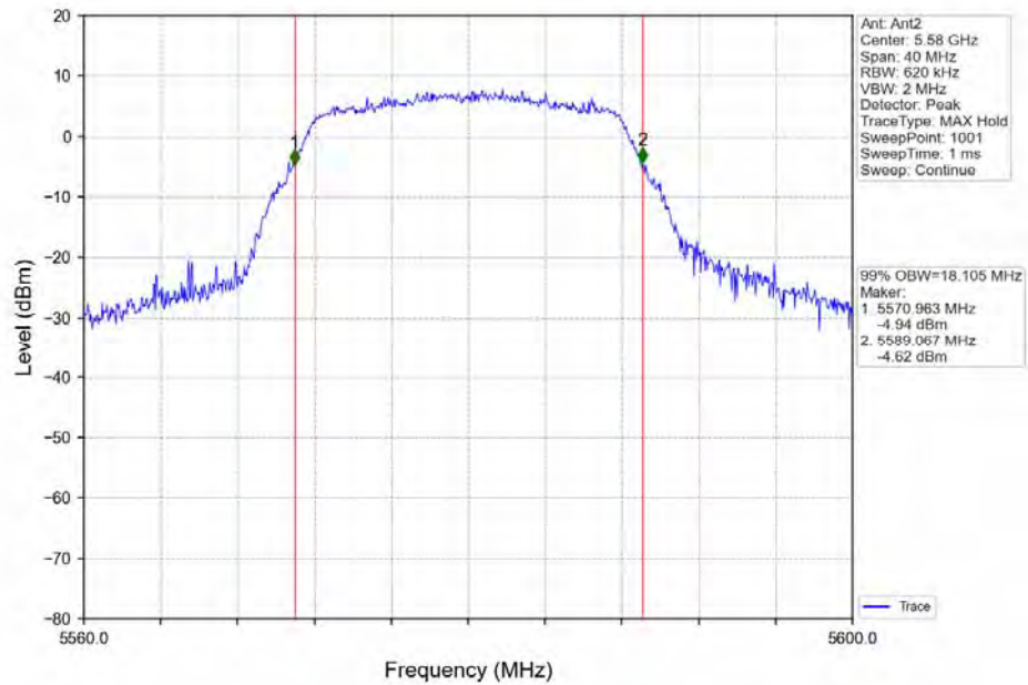
802.11a_MCH_5580MHz_Ant2_NTNV
