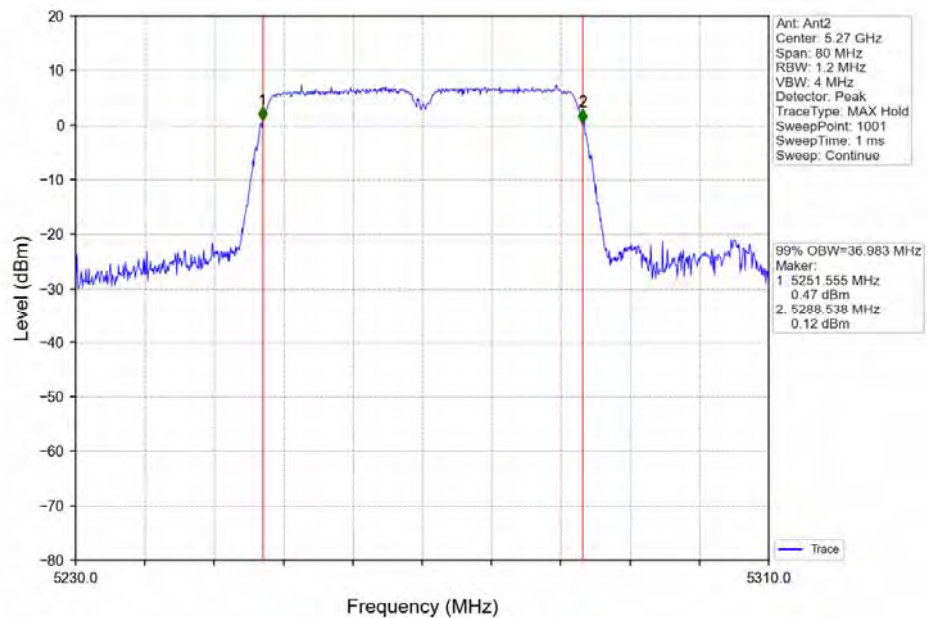
802.11n(HT40) LCH_5270MHz_Ant2_NTNV
