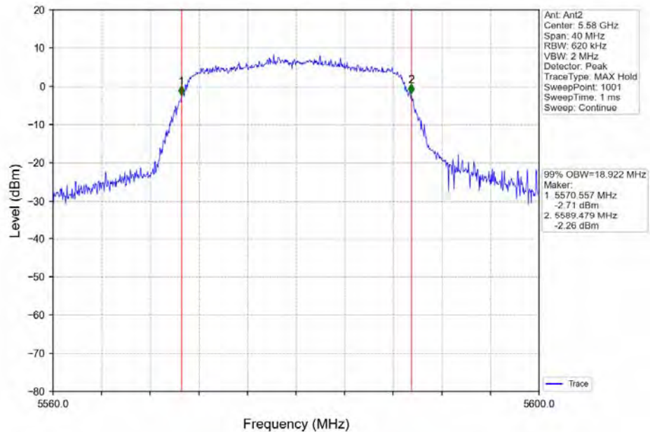
802.11n(HT20) MCH_5580MHz_Ant2_NTNV
