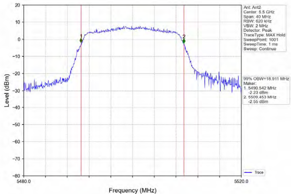
802.11n(HT20) LCH_5500MHz_Ant2_NTNV
