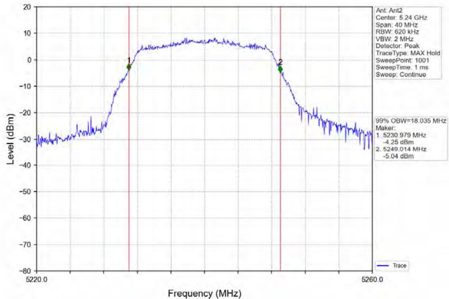
802.11a_HCH_5240MHz_Ant2_NTNV
