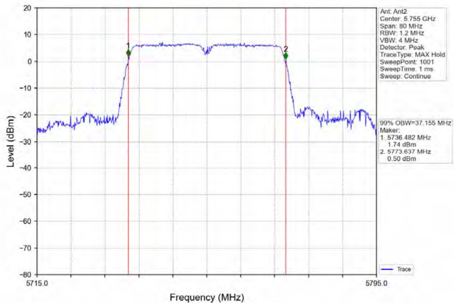
802.11n(HT40) LCH_5755MHz_Ant2_NTNV
