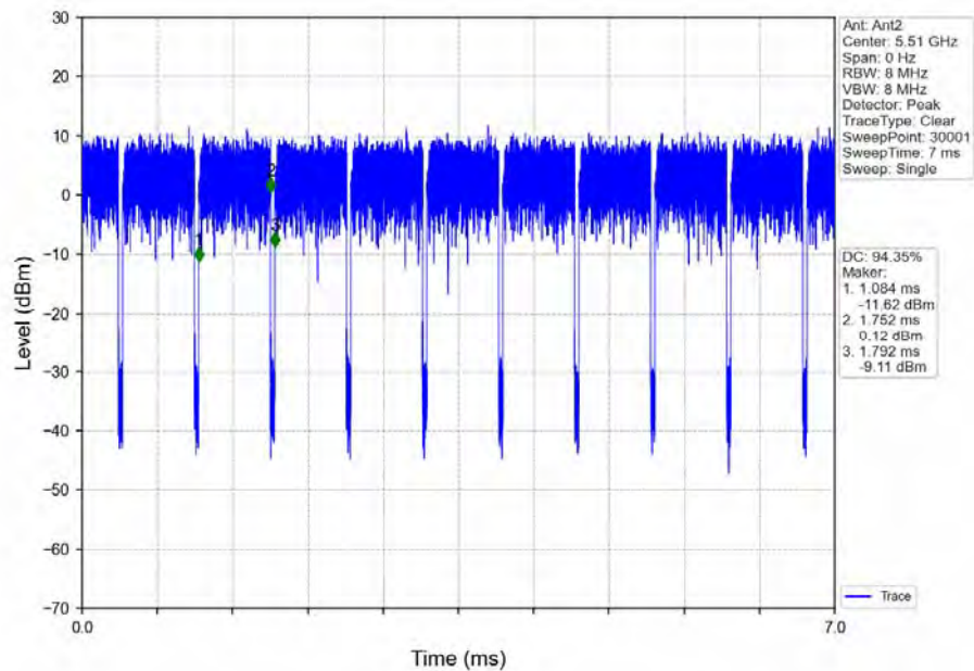
802.11ac(VHT40) LCH_5510MHz_Ant2_NTNV
