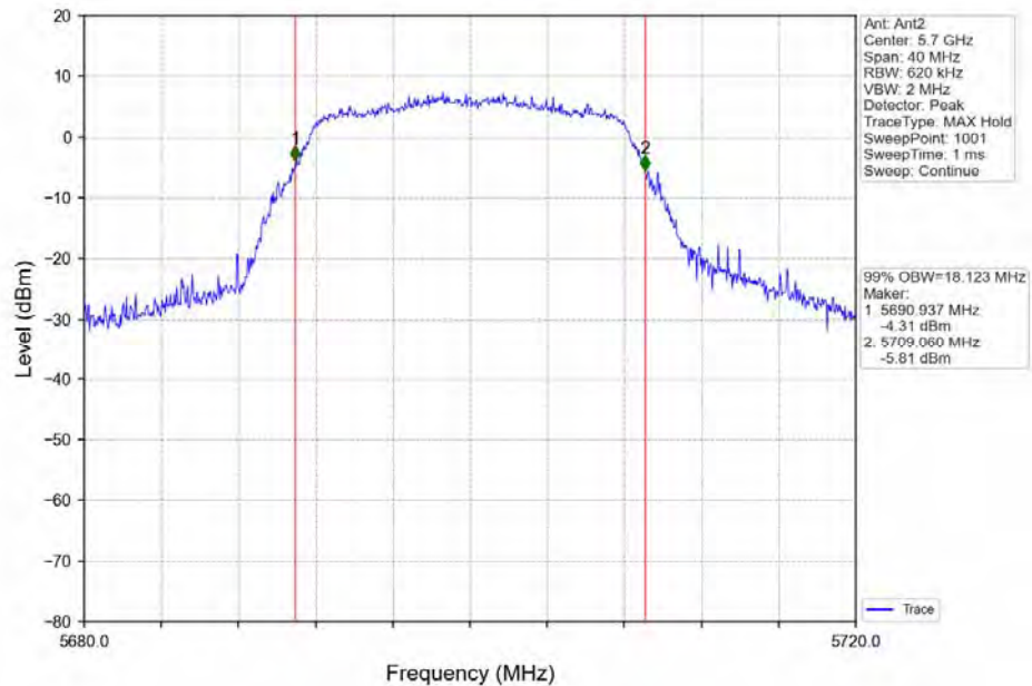
802.11a_HCH_5700MHz_Ant2_NTNV
