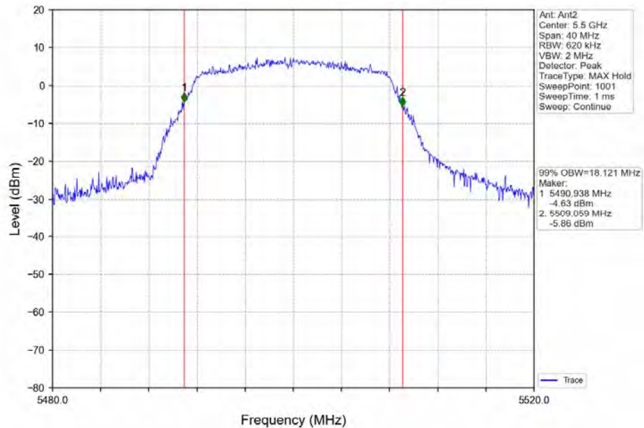
802.11a_LCH_5500MHz_Ant2_NTNV
