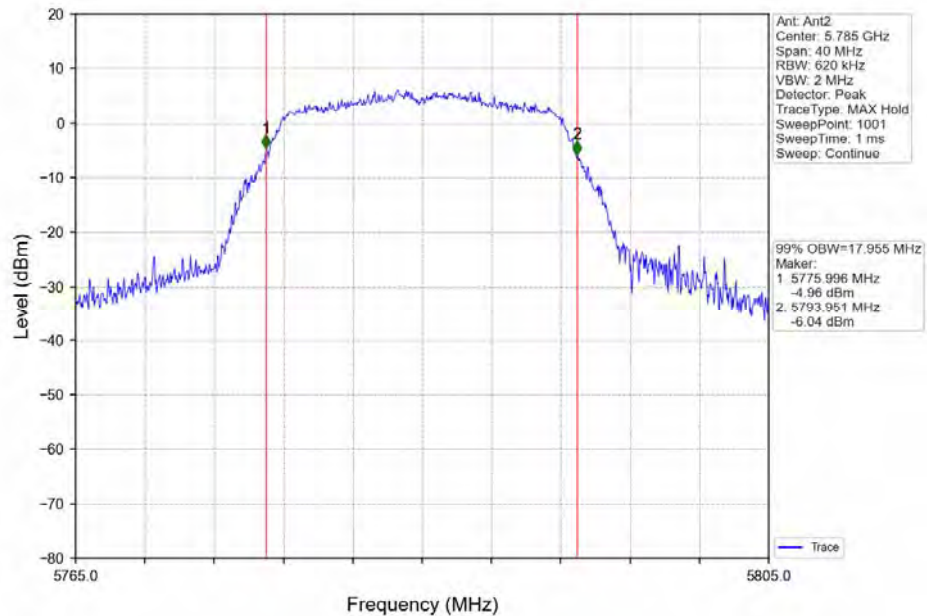
802.11a_MCH_5785MHz_Ant2_NTNV
