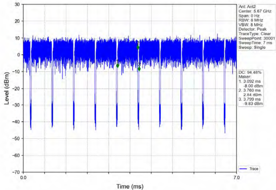
802.11ac(VHT40) HCH_5670MHz_Ant2_NTNV
