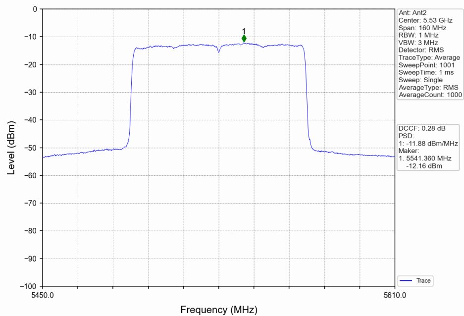
802.11ax(HEW80)_LCH_5530MHz_Ant2_NTNV
