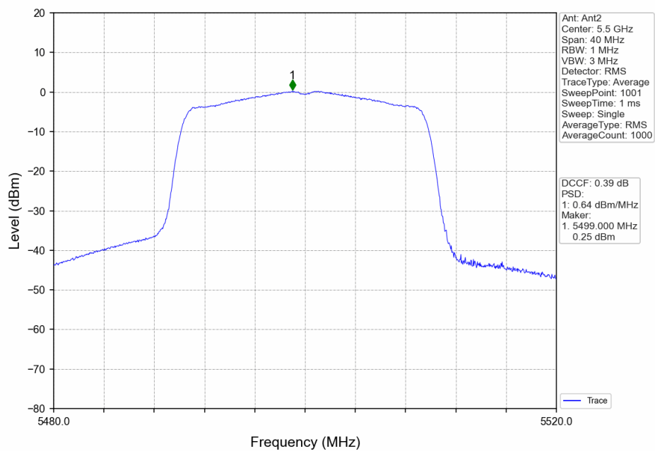
802.11ax(HEW20)_LCH_5500MHz_Ant2_NTNV
