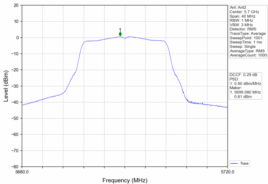
802.11a_HCH_5700MHz_Ant2_NTNV
