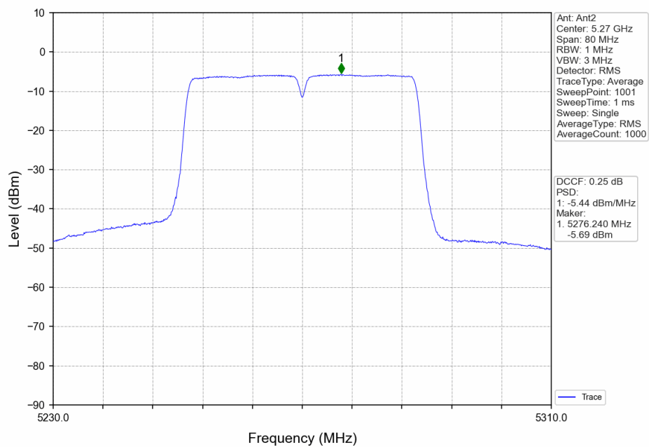
802.11ac(VHT40)_LCH_5270MHz_Ant2_NTNV
