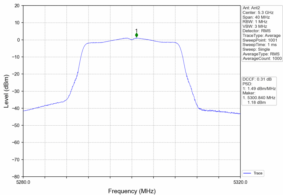
802.11n(HT20)_MCH_5300MHz_Ant2_NTNV
