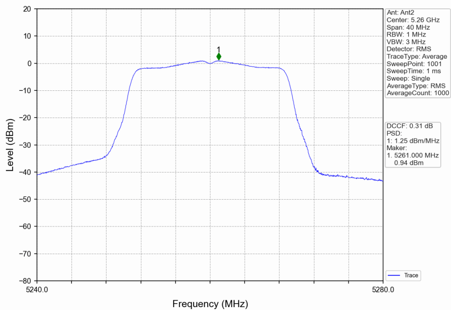
802.11n(HT20)_LCH_5260MHz_Ant2_NTNV
