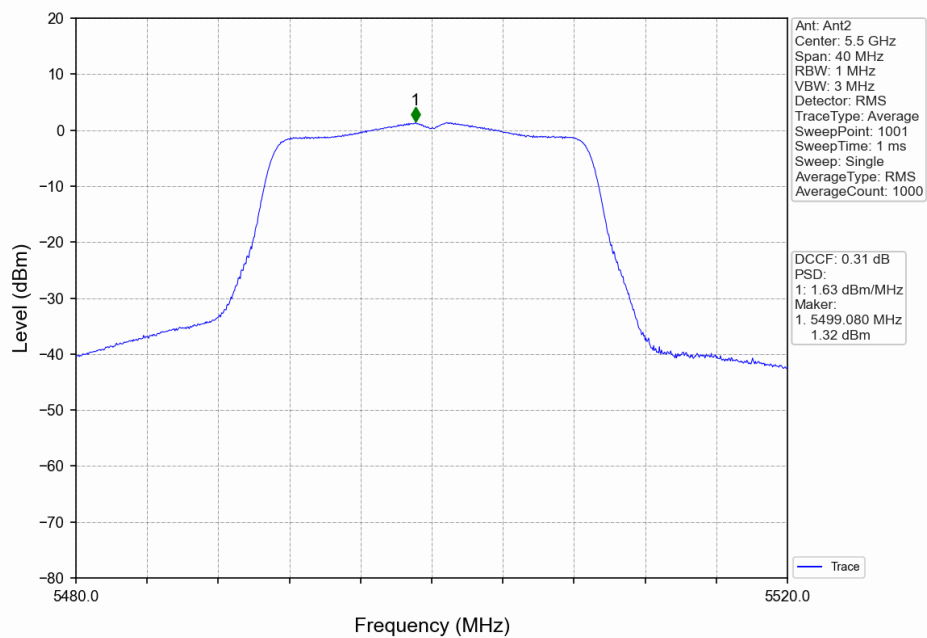
802.11n(HT20)_LCH_5500MHz_Ant2_NTNV
