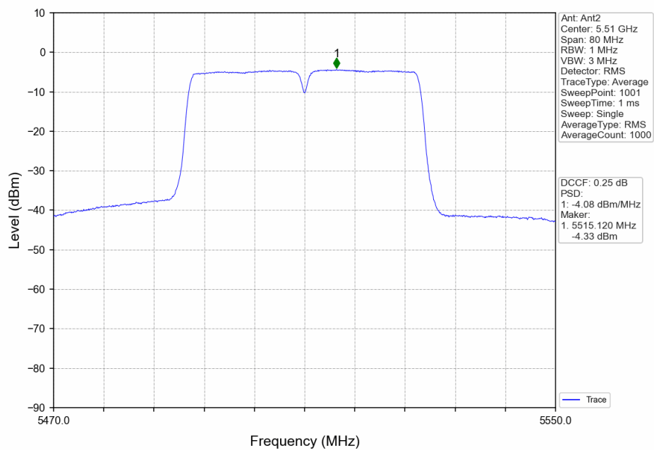
802.11n(HT40)_LCH_5510MHz_Ant2_NTNV
