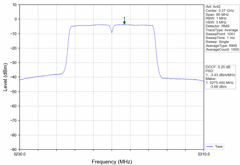
802.11n(HT40)_LCH_5270MHz_Ant2_NTNV
