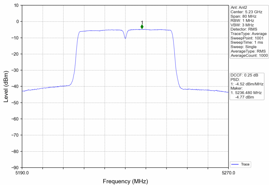
802.11n(HT40)_HCH_5230MHz_Ant2_NTNV
