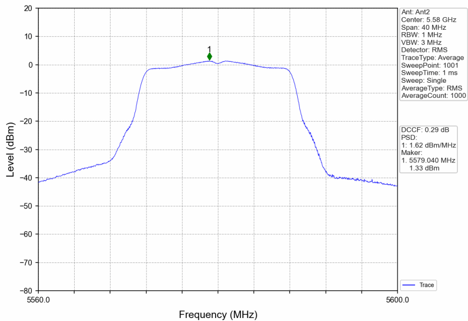
802.11a_MCH_5580MHz_Ant2_NTNV
