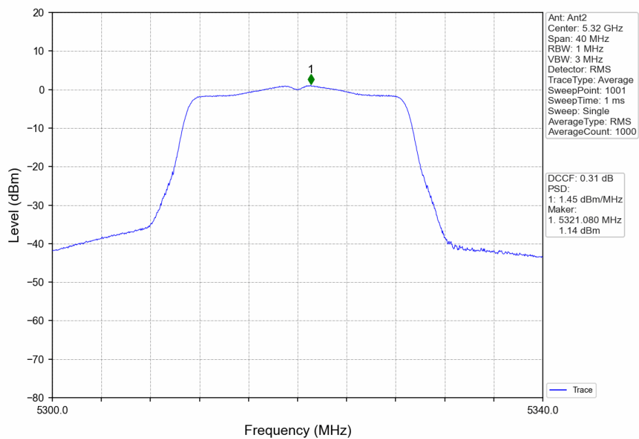
802.11n(HT20)_HCH_5320MHz_Ant2_NTNV
