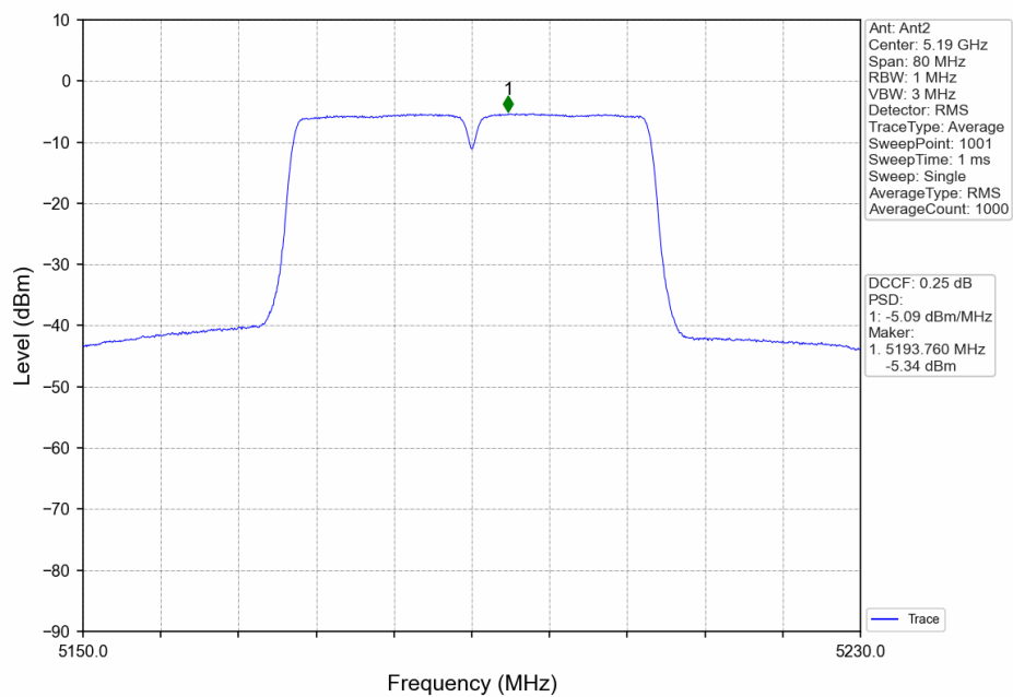
802.11n(HT40)_LCH_5190MHz_Ant2_NTNV
