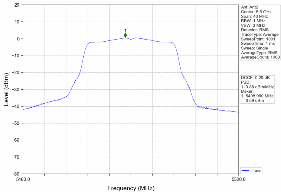
802.11a_LCH_5500MHz_Ant2_NTNV
