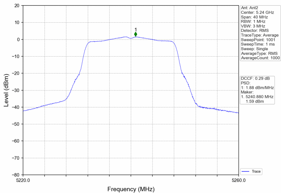
802.11a_HCH_5240MHz_Ant2_NTNV
