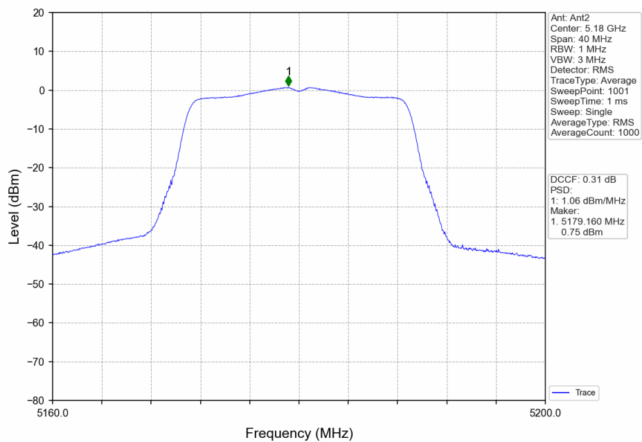
802.11n(HT20)_LCH_5180MHz_Ant2_NTNV
