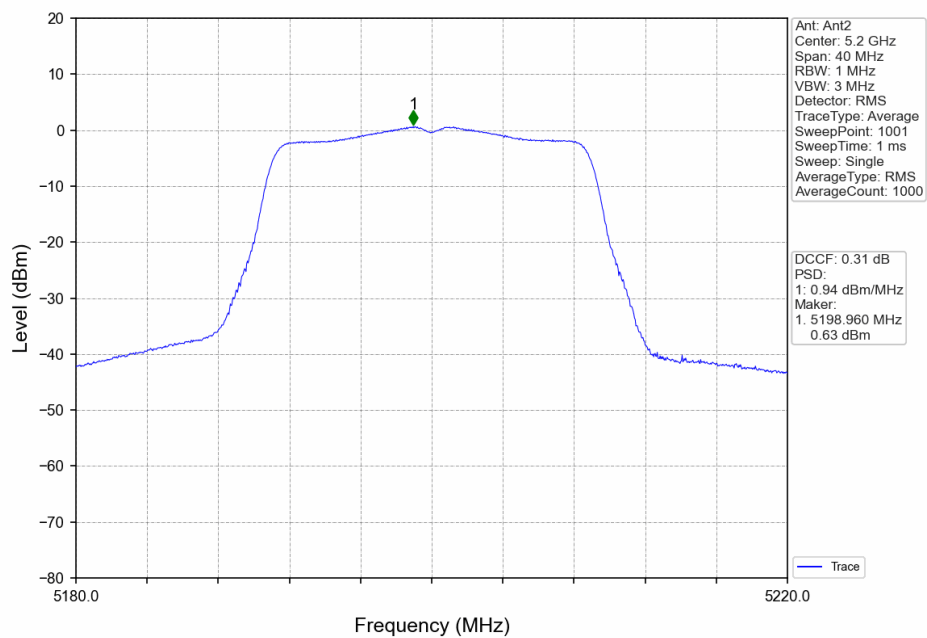
802.11n(HT20)_MCH_5200MHz_Ant2_NTNV
