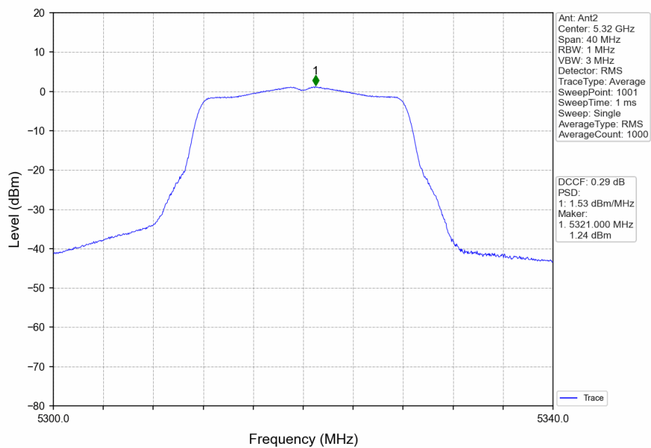
802.11a_HCH_5320MHz_Ant2_NTNV
