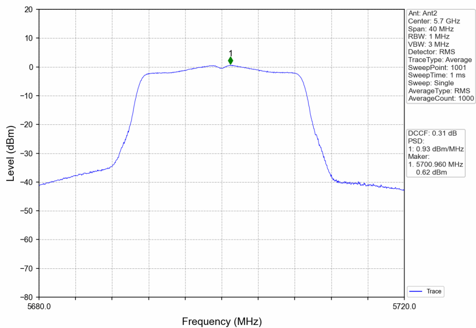
802.11n(HT20)_HCH_5700MHz_Ant2_NTNV
