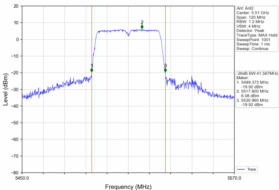
802.11n(HT40)_LCH_5510MHz_Ant2_NTNV
