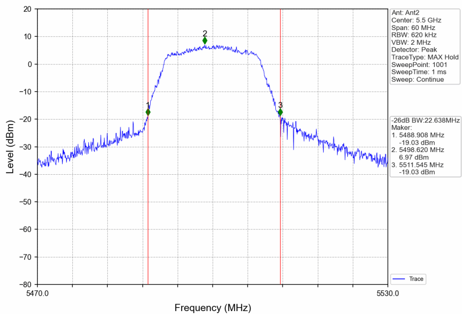
802.11a_LCH_5500MHz_Ant2_NTNV
