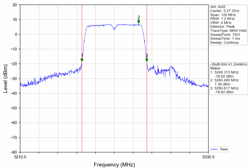
802.11n(HT40)_LCH_5270MHz_Ant2_NTNV
