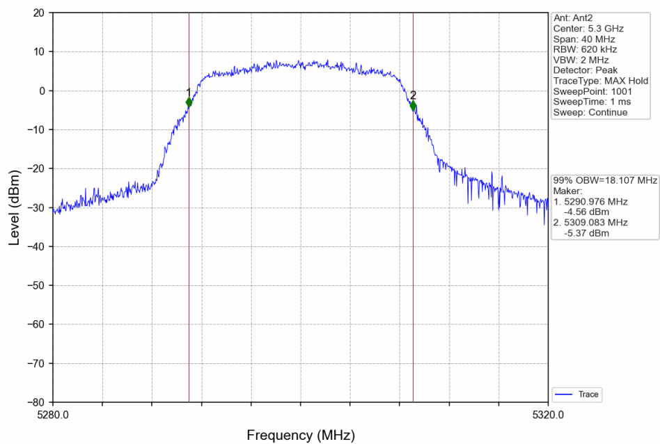
802.11a_MCH_5300MHz_Ant2_NTNV
