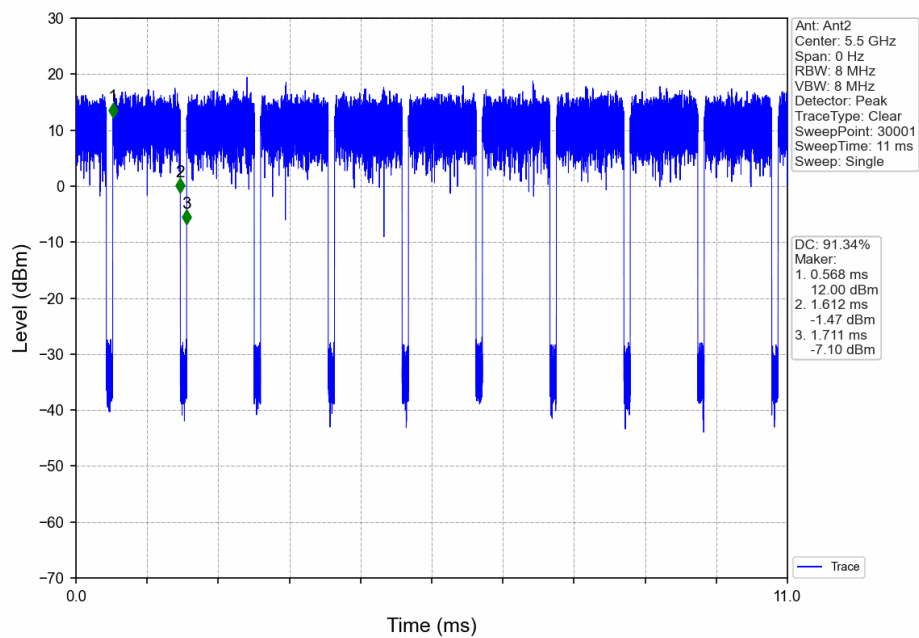
802.11ax(HEW20)_LCH_5500MHz_Ant2_NTNV
