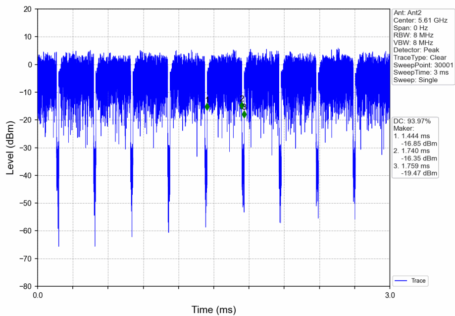
802.11ax(HEW80)_HCH_5610MHz_Ant2_NTNV
