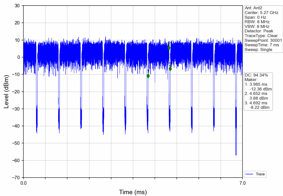
802.11ac(VHT40)_LCH_5270MHz_Ant2_NTNV
