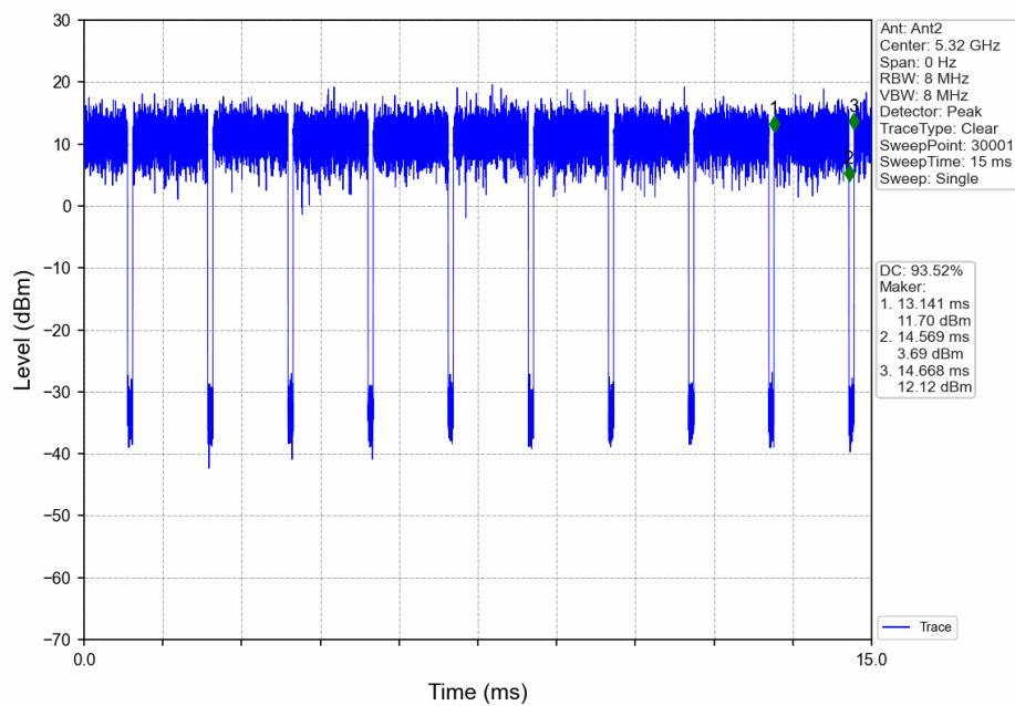
802.11a_HCH_5320MHz_Ant2_NTNV
