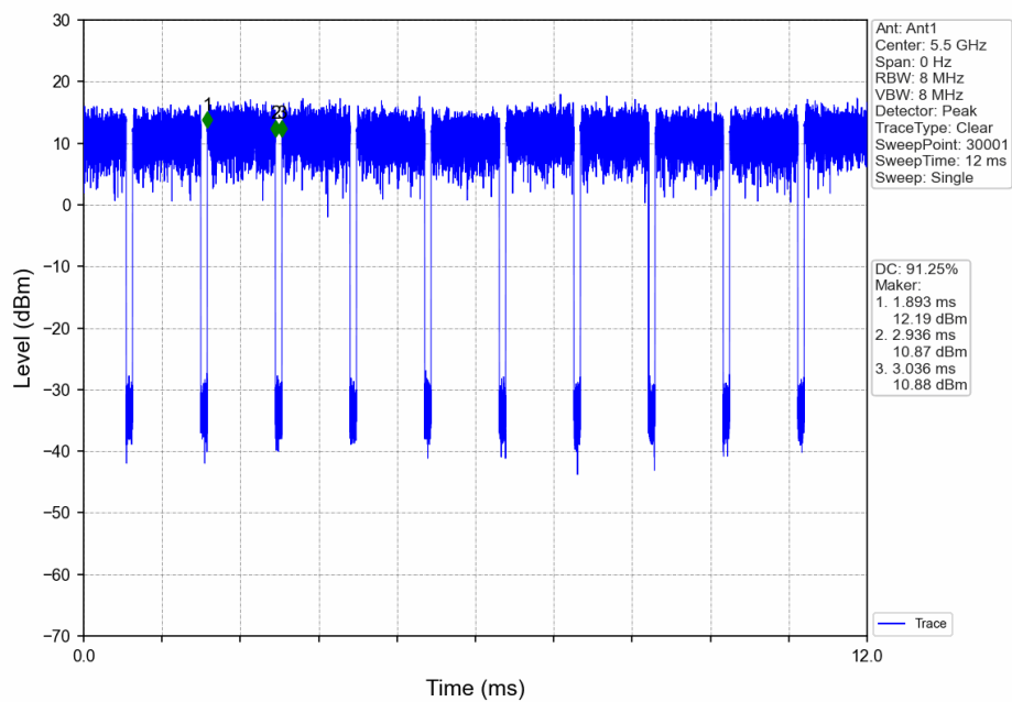
802.11ax(HEW20)_LCH_5500MHz_Ant1_NTNV
