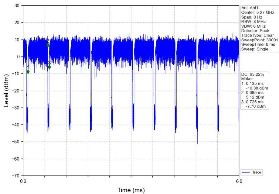
802.11ax(HEW40)_LCH_5270MHz_Ant1_NTNV
