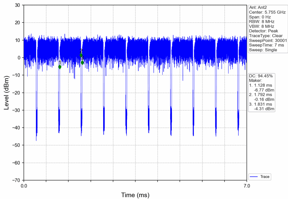
802.11n(HT40)_LCH_5755MHz_Ant2_NTNV
